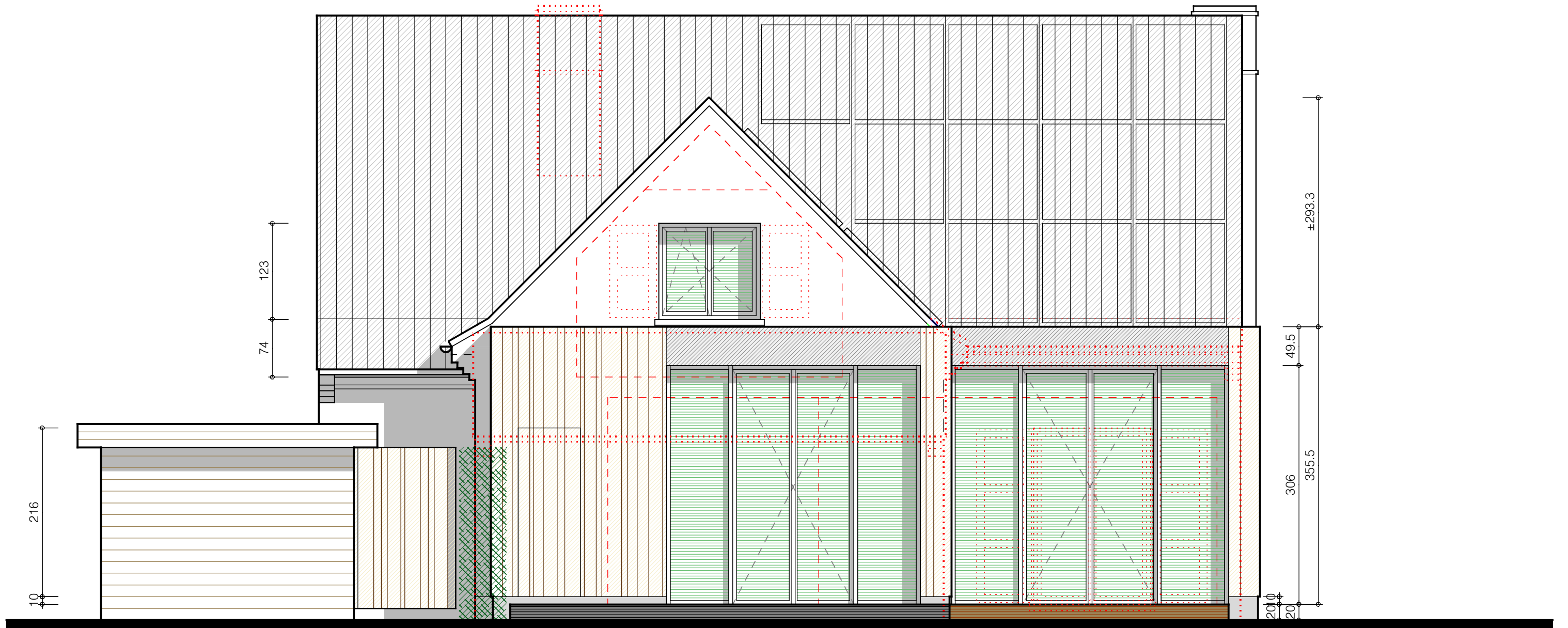
achtergevel west
