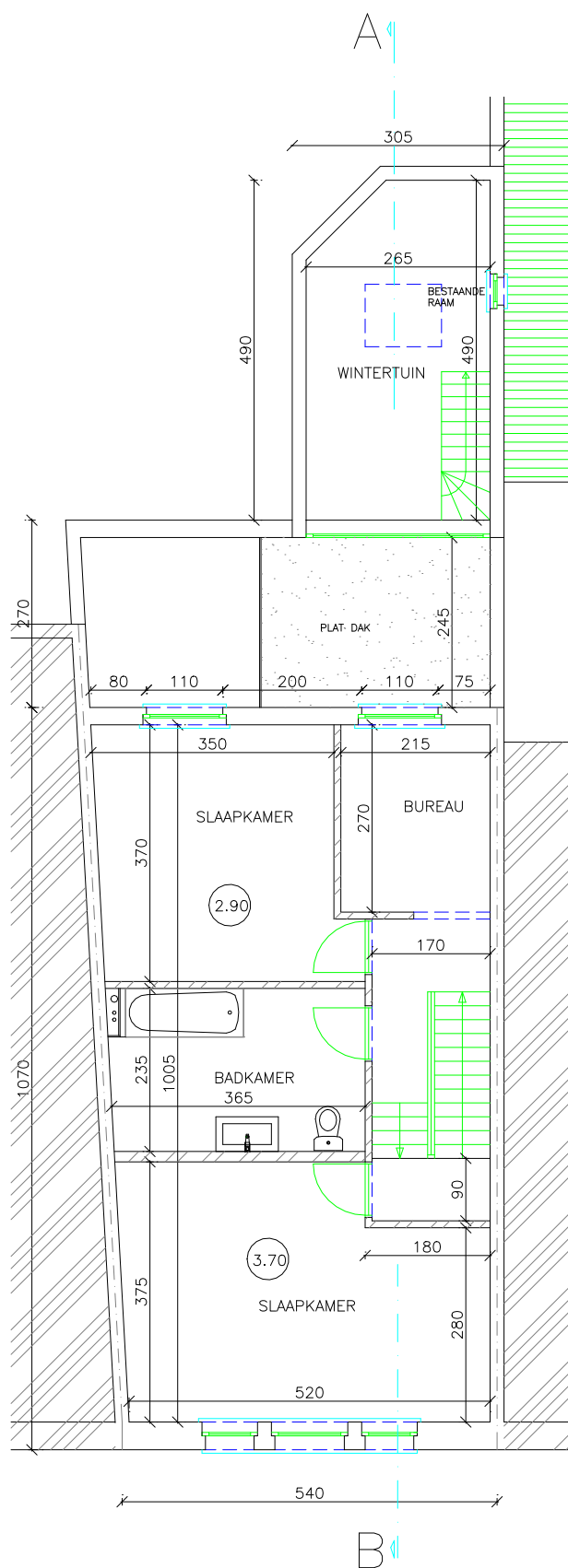
BA woning-P-V-2-verdieping 1
