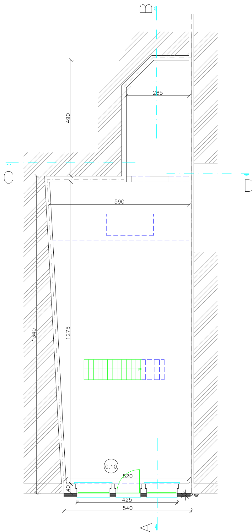
BA woning-P-B-1-gelijkvloers
