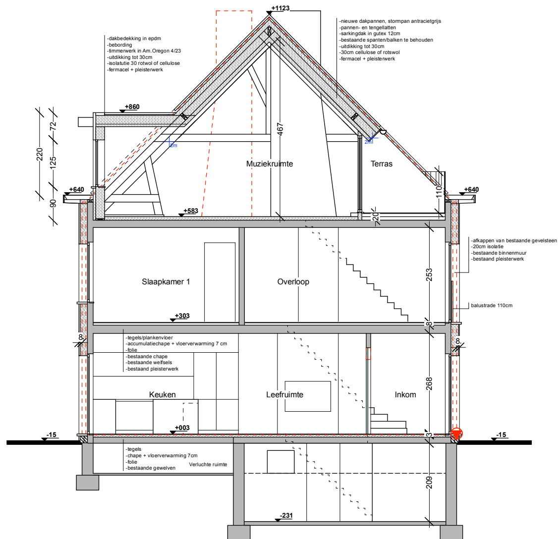
EB 1240: DOORSNEDE AA nieuwe toestand 1/100
