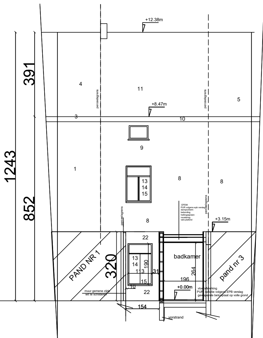
DOORSNEDE CD en ACHTERGEVEL 1/100
