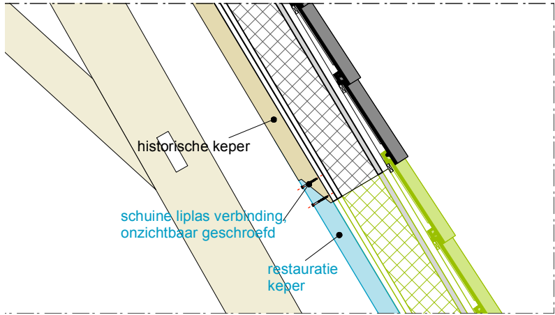
Situatie 1: schuine liplas verbinding
