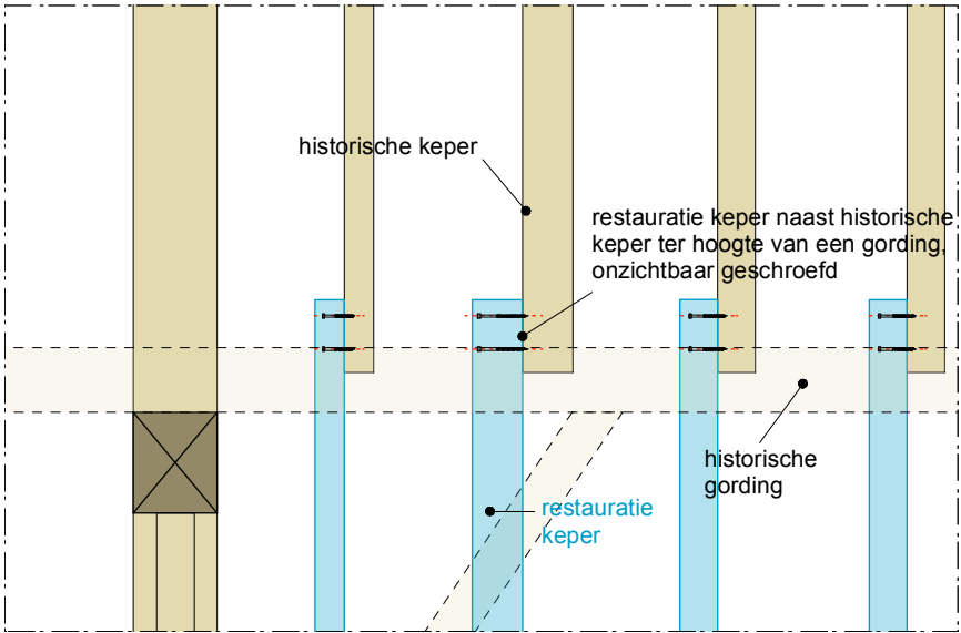
Situatie 2: kepers naast elkaar
