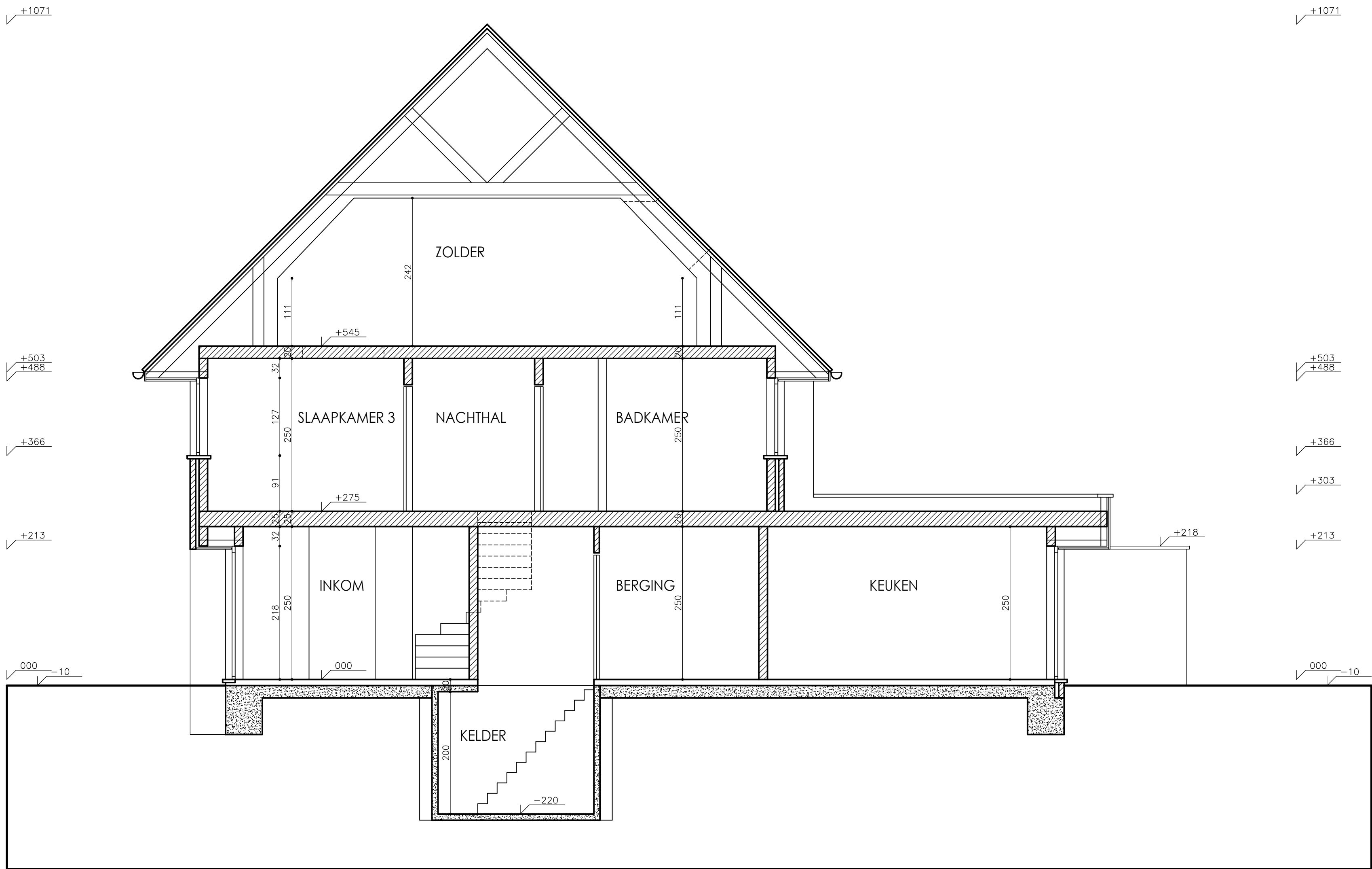
DOORSNEDE AB
