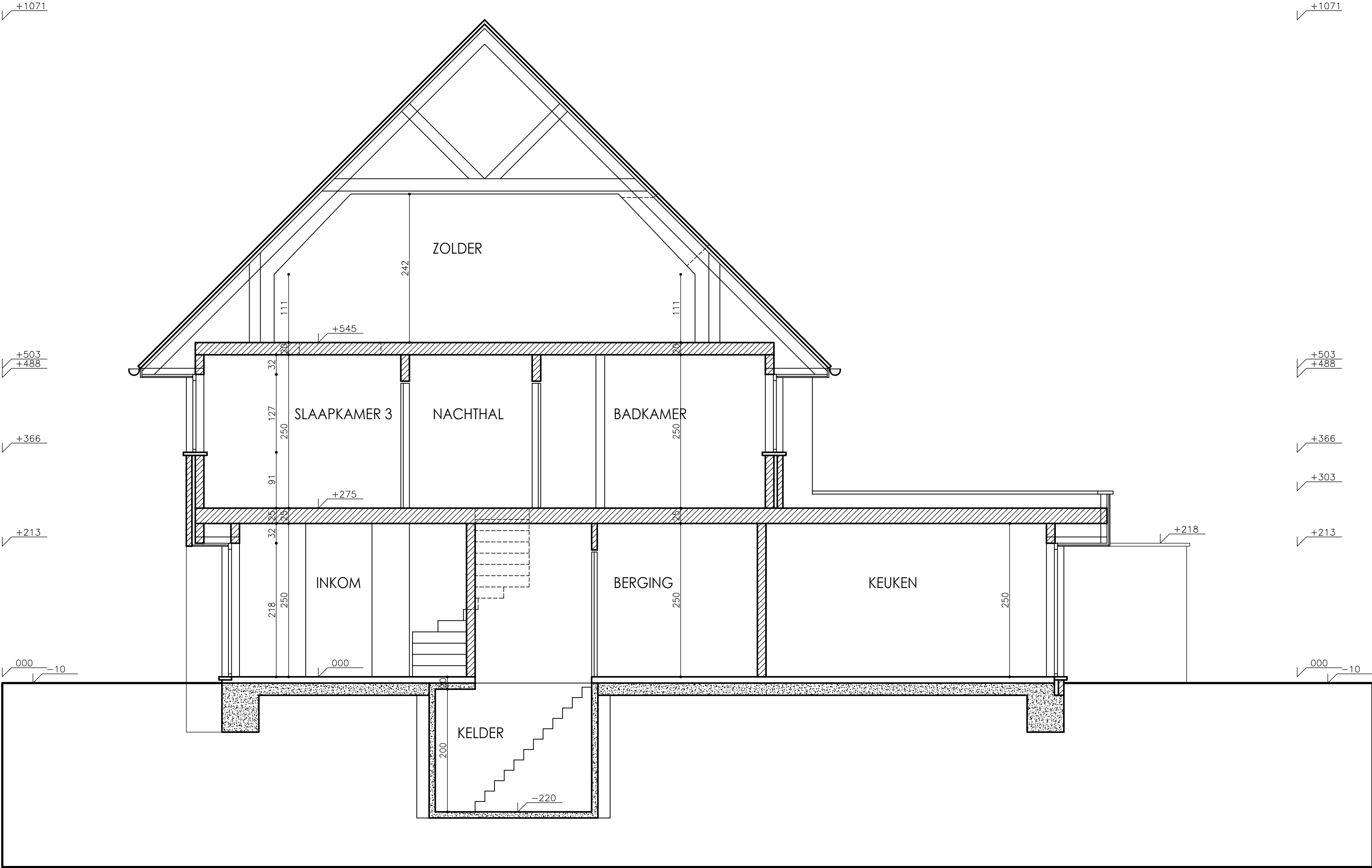
DOORSNEDE AB
