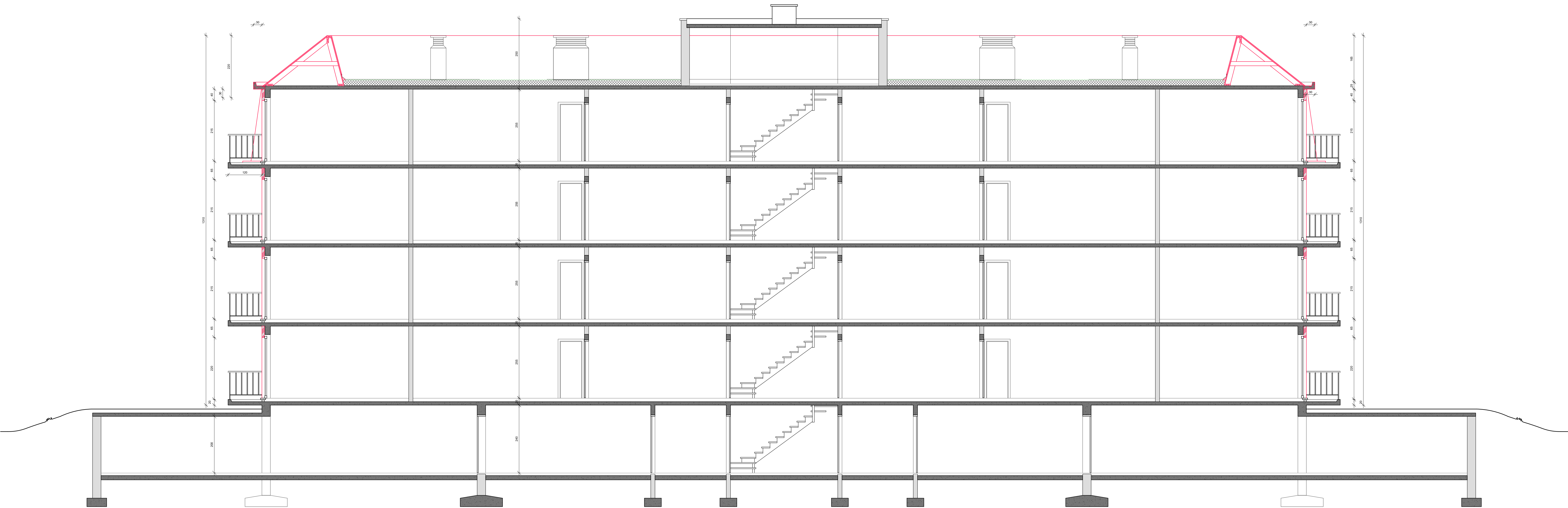
BT LANGSDOORSNEDE
