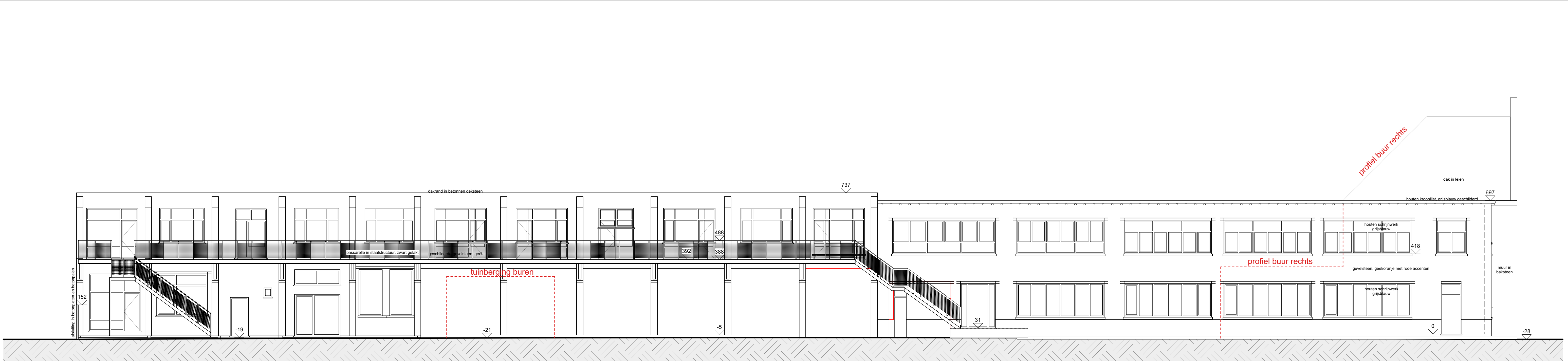
Linker zijgevelaanzicht nieuwe toestand
