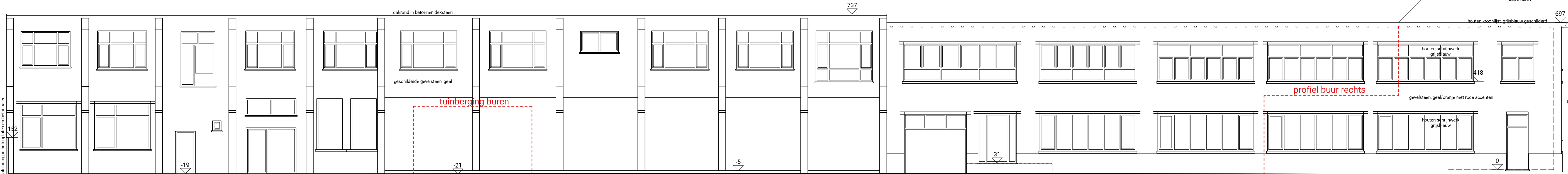
schaal: 1:100
