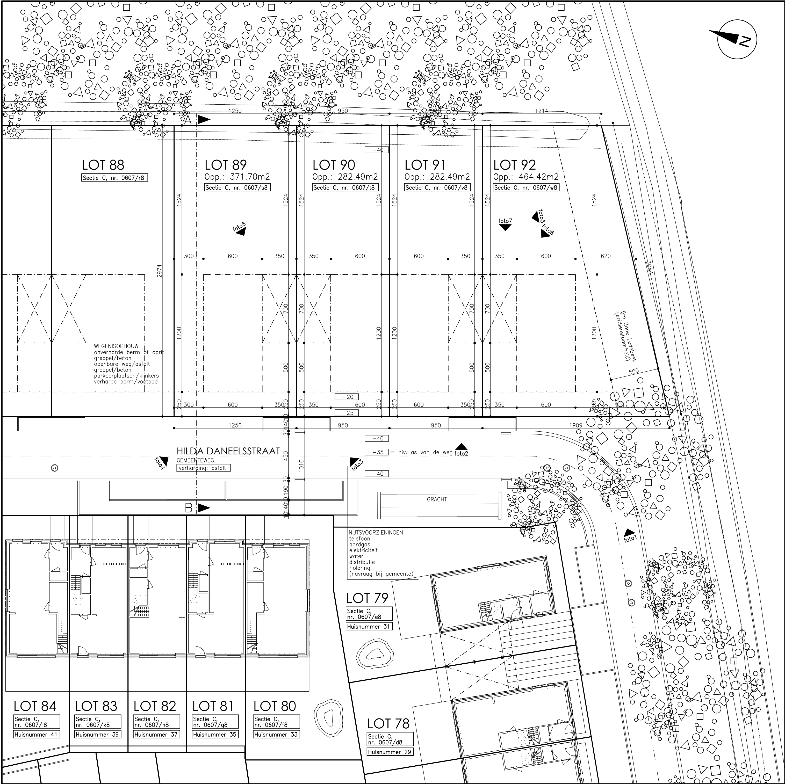
INPLANTING - BESTAANDE TOESTAND
