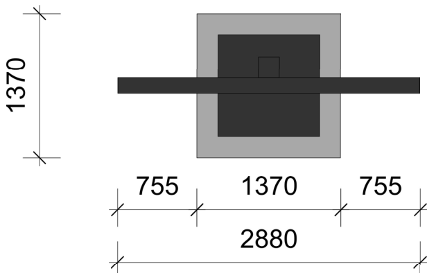
Bovenaanzicht scherm
