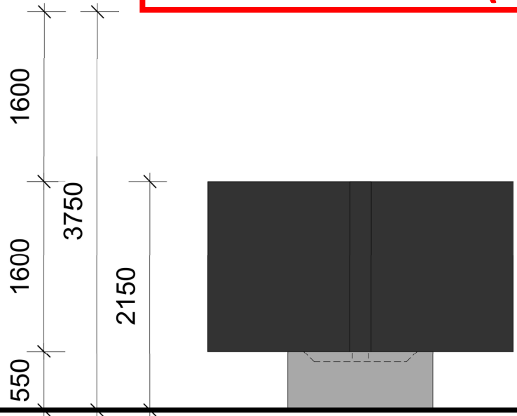
Achterzijde scherm: minimale hoogte
