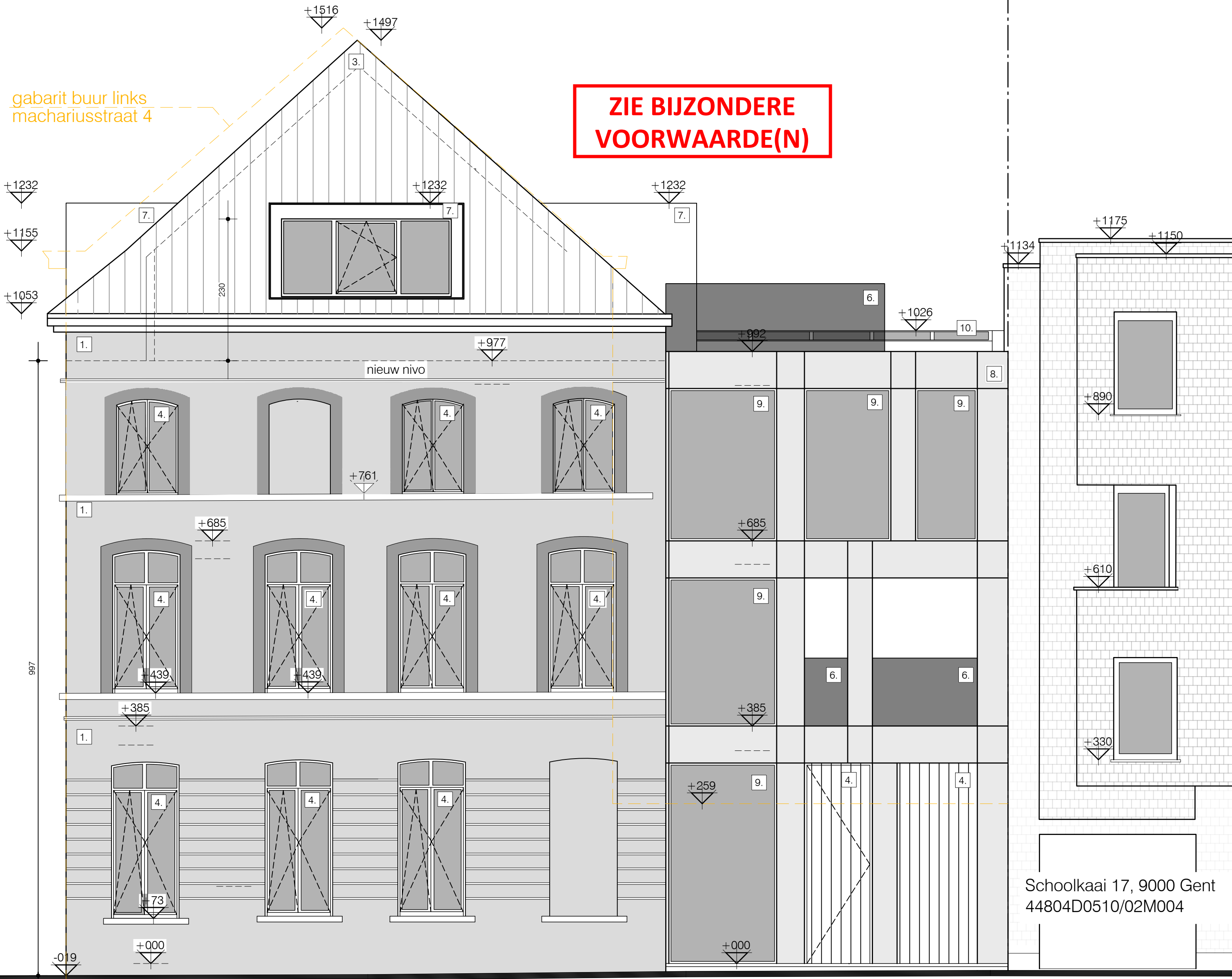
NIEUWE TOESTAND VOORGEVEL (Schoolkaai) schaal: 1/50 - maatvoering in cm
