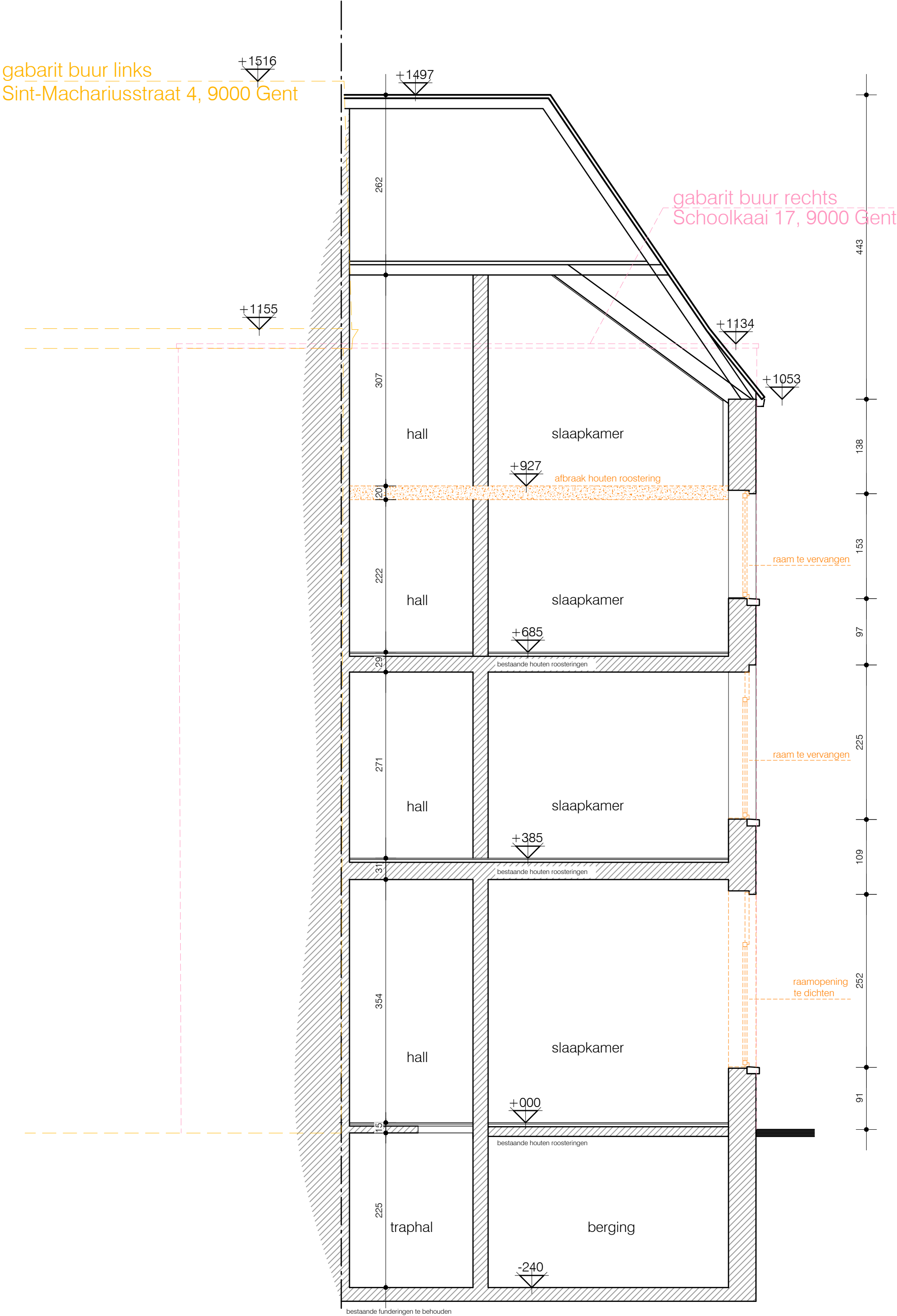
BESTAANDE TOESTAND SNEDE A-A schaal: 1/50 - maatvoering in cm
