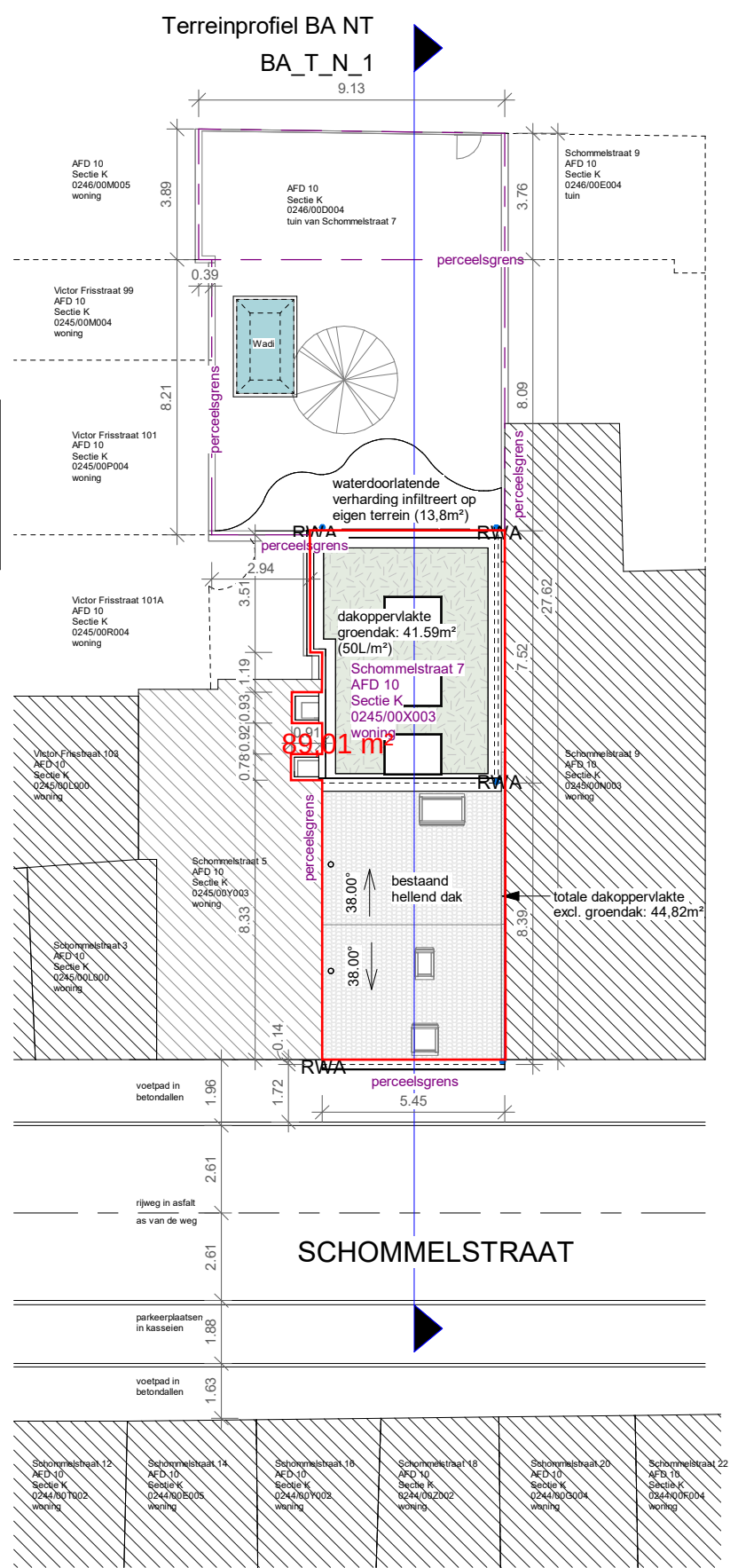
1 1 : 200 Inplantingsplan nieuwe toestand
