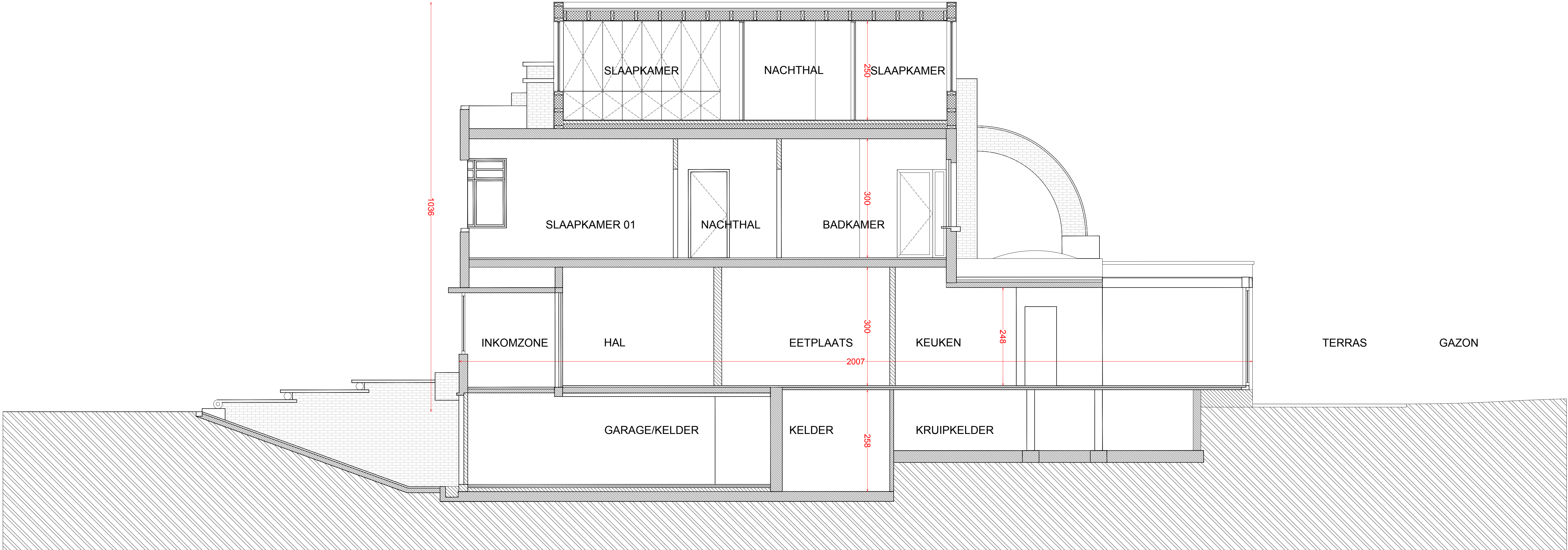
SINT-DENIJSLAAN 102 - GENT SNEDE A - SCHAAL 1:50 NIEUWE TOESTAND
