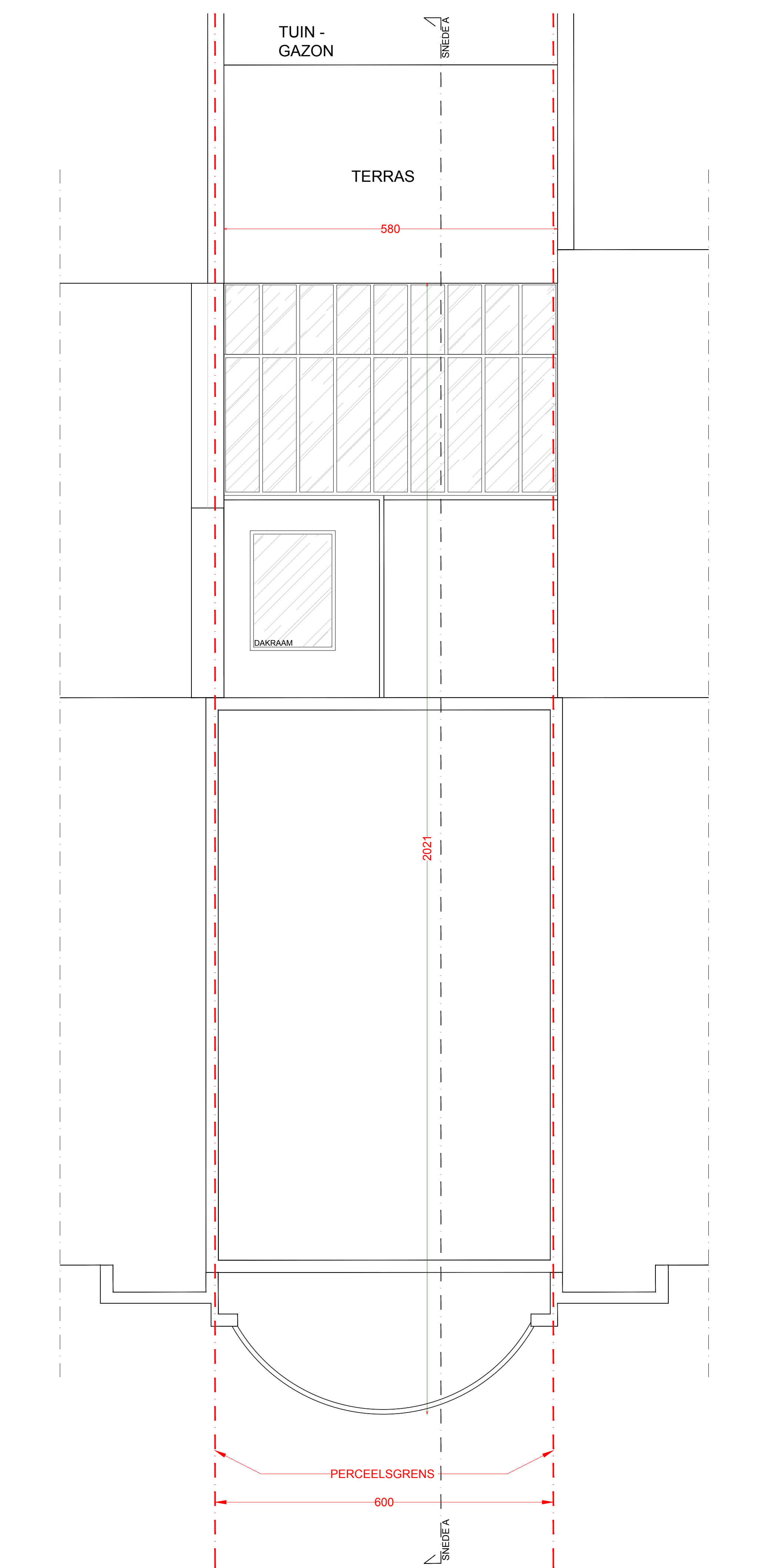
SINT-DENIJSLAAN 102 - GENT DAKENPLAN - SCHAAL 1:50 NIEUWE TOESTAND
