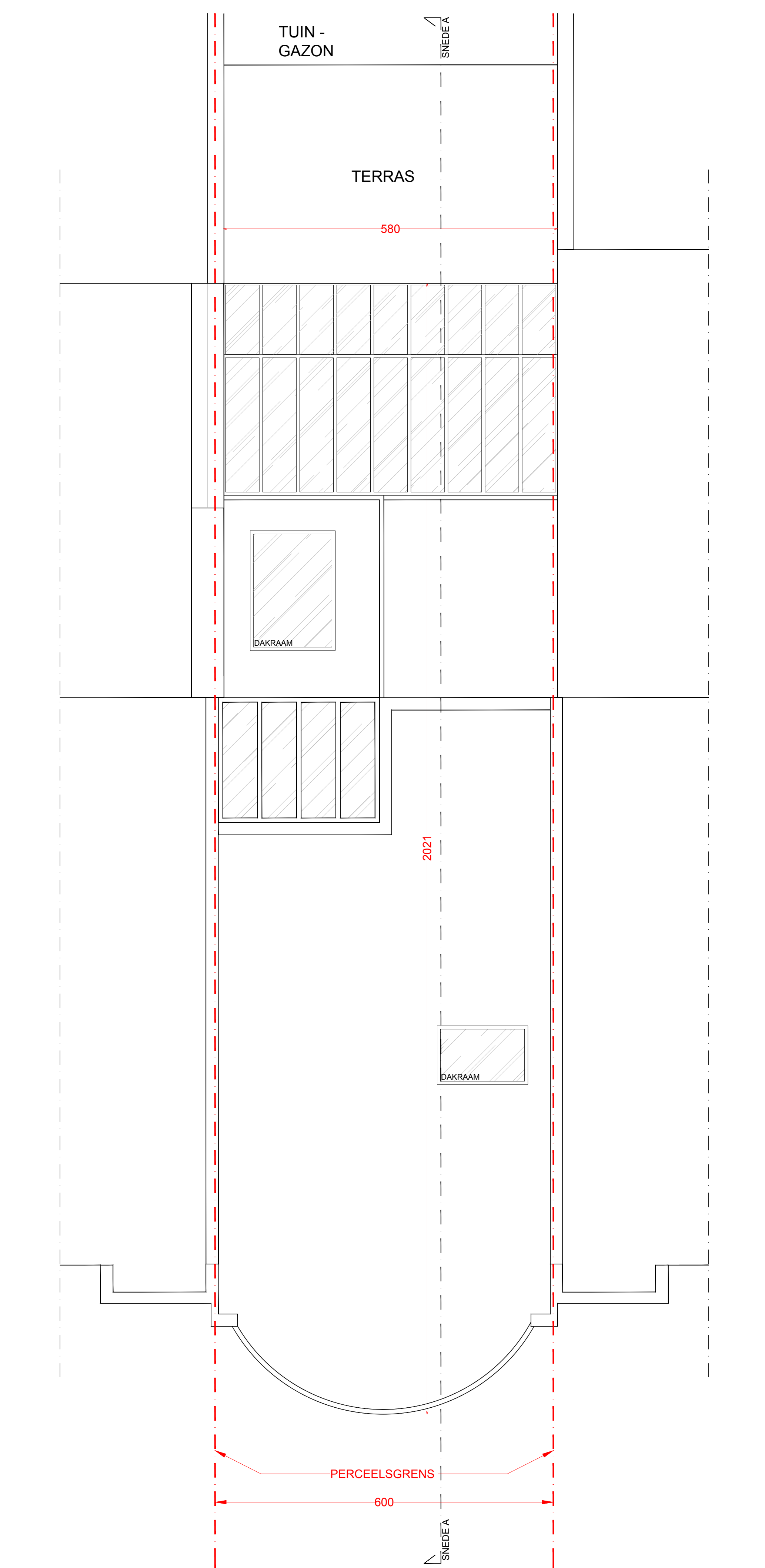
SINT-DENIJSLAAN 102 - GENT DAKENPLAN - SCHAAL 1:50 BESTAANDE TOESTAND
