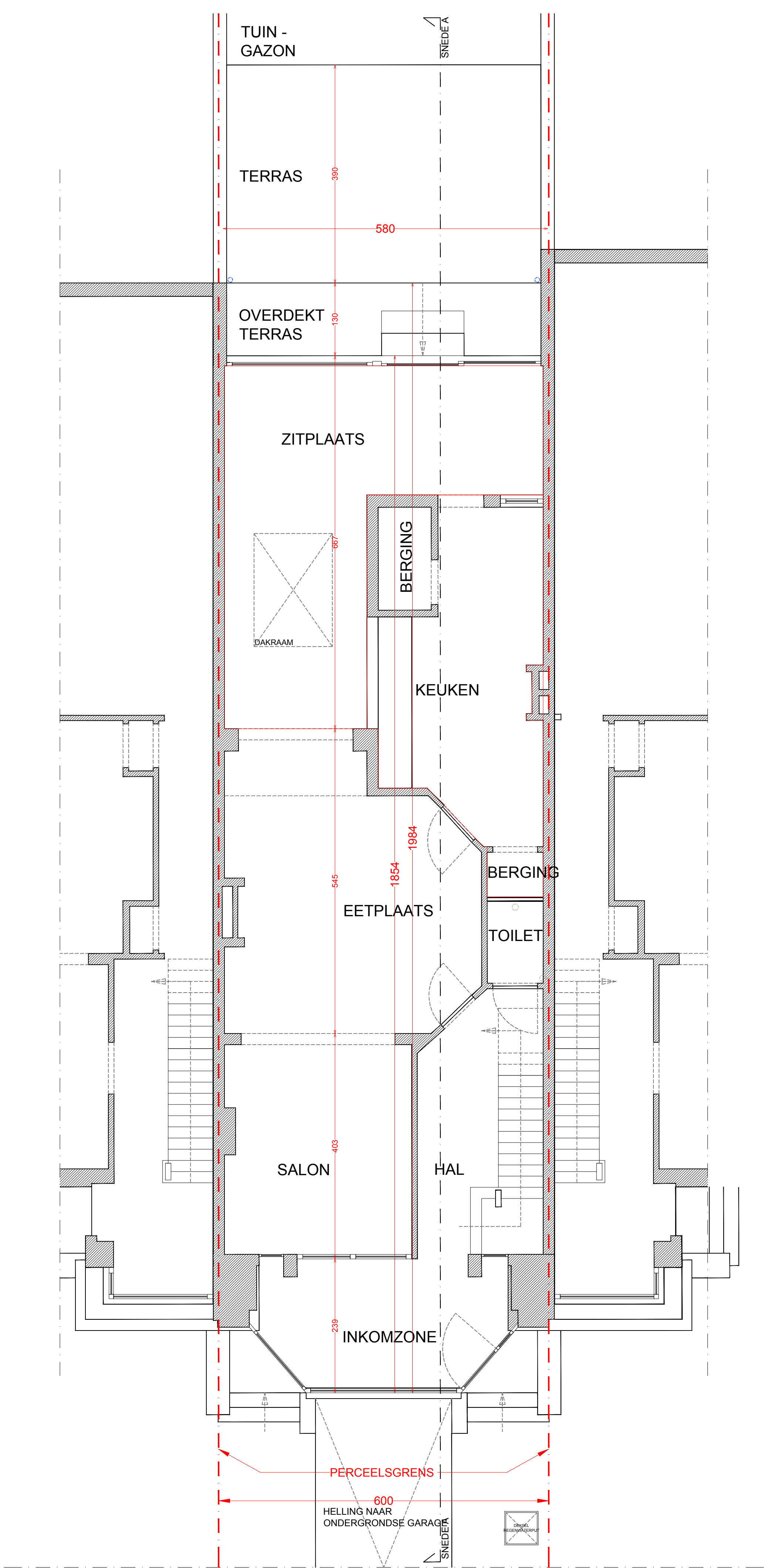
SINT-DENIJSLAAN 102 - GENT PLAN GELIJKVLOERS - SCHAAAL 1:50 BESTAANDE TOESTAND
