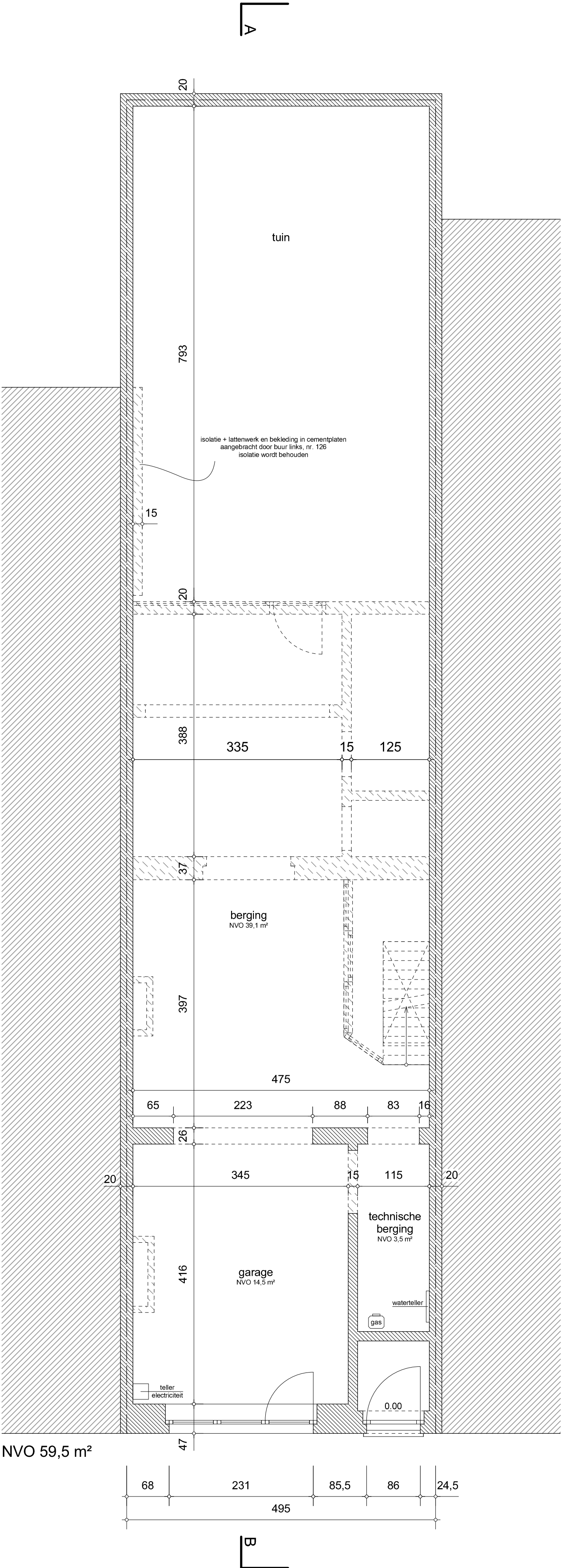
GRONDPLAN NIVO 0 BESTAANDE TOESTAND schaal 1/50
