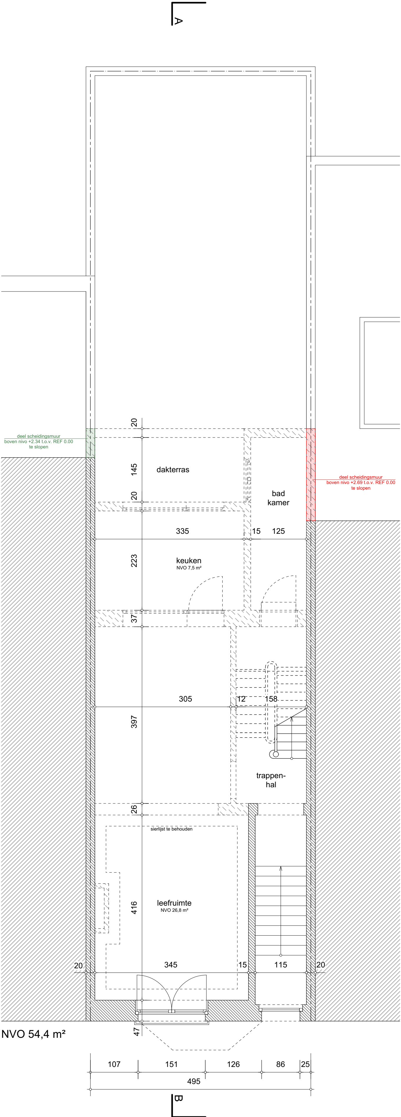
GRONDPLAN NIVO +1 BESTAANDE TOESTAND schaal 1/50
