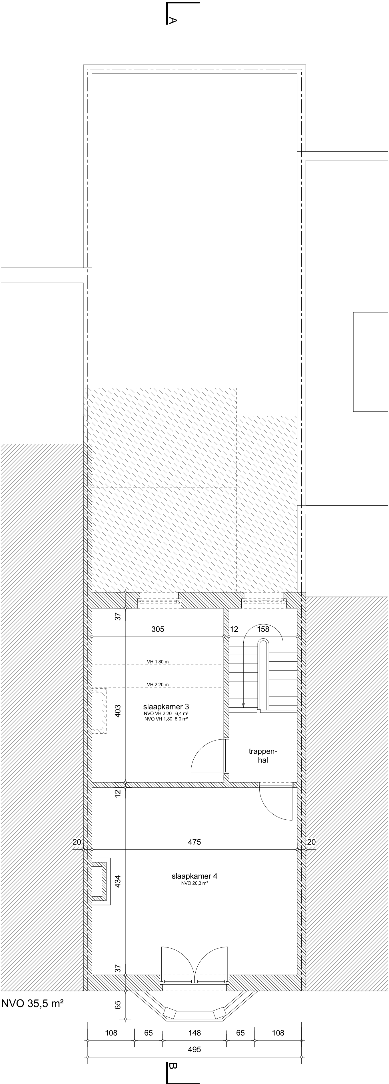
GRONDPLAN NIVO +3 BESTAANDE TOESTAND schaal 1/50
