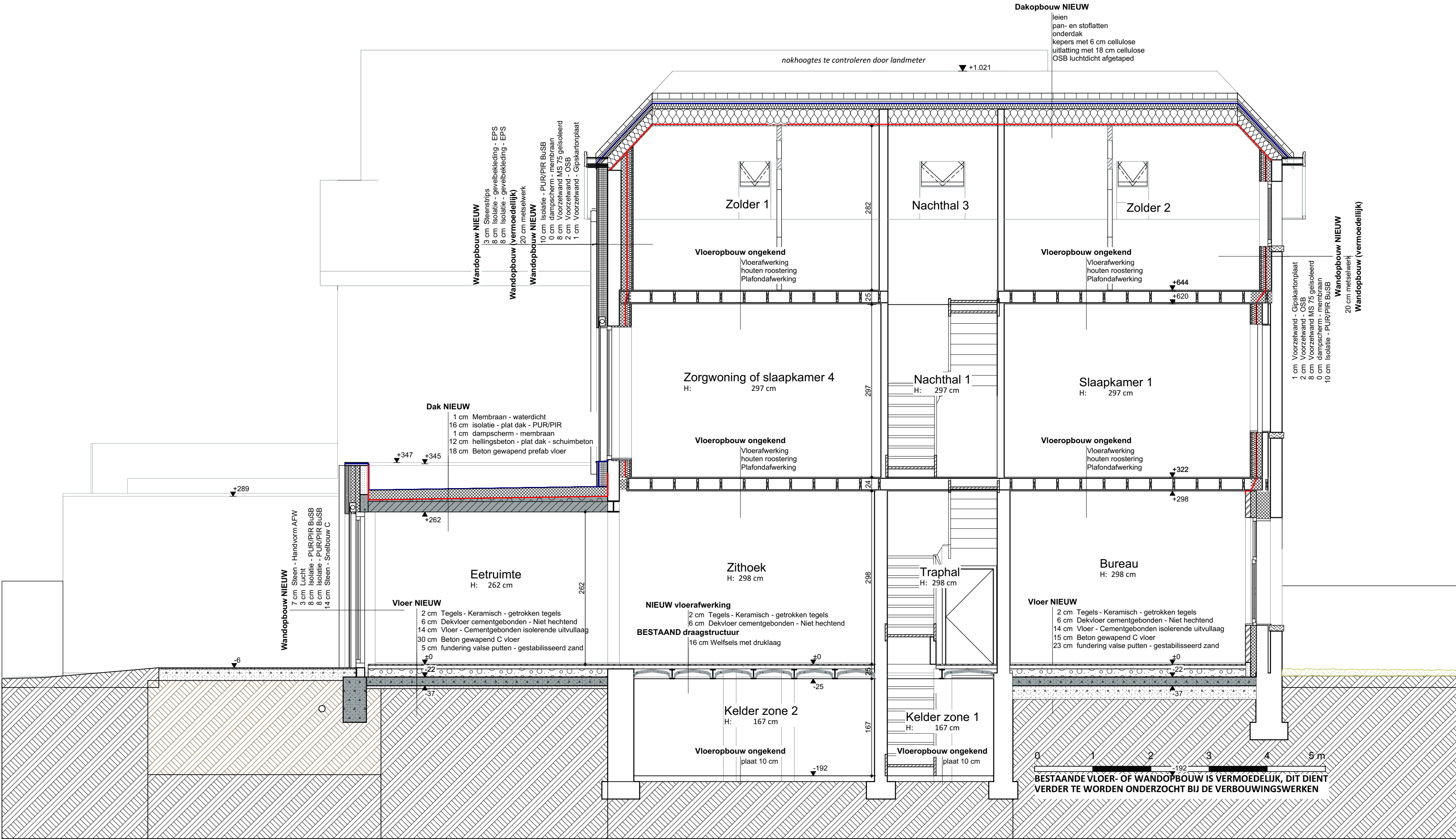
DOORSNEDE S4 - Nieuwe toestand
