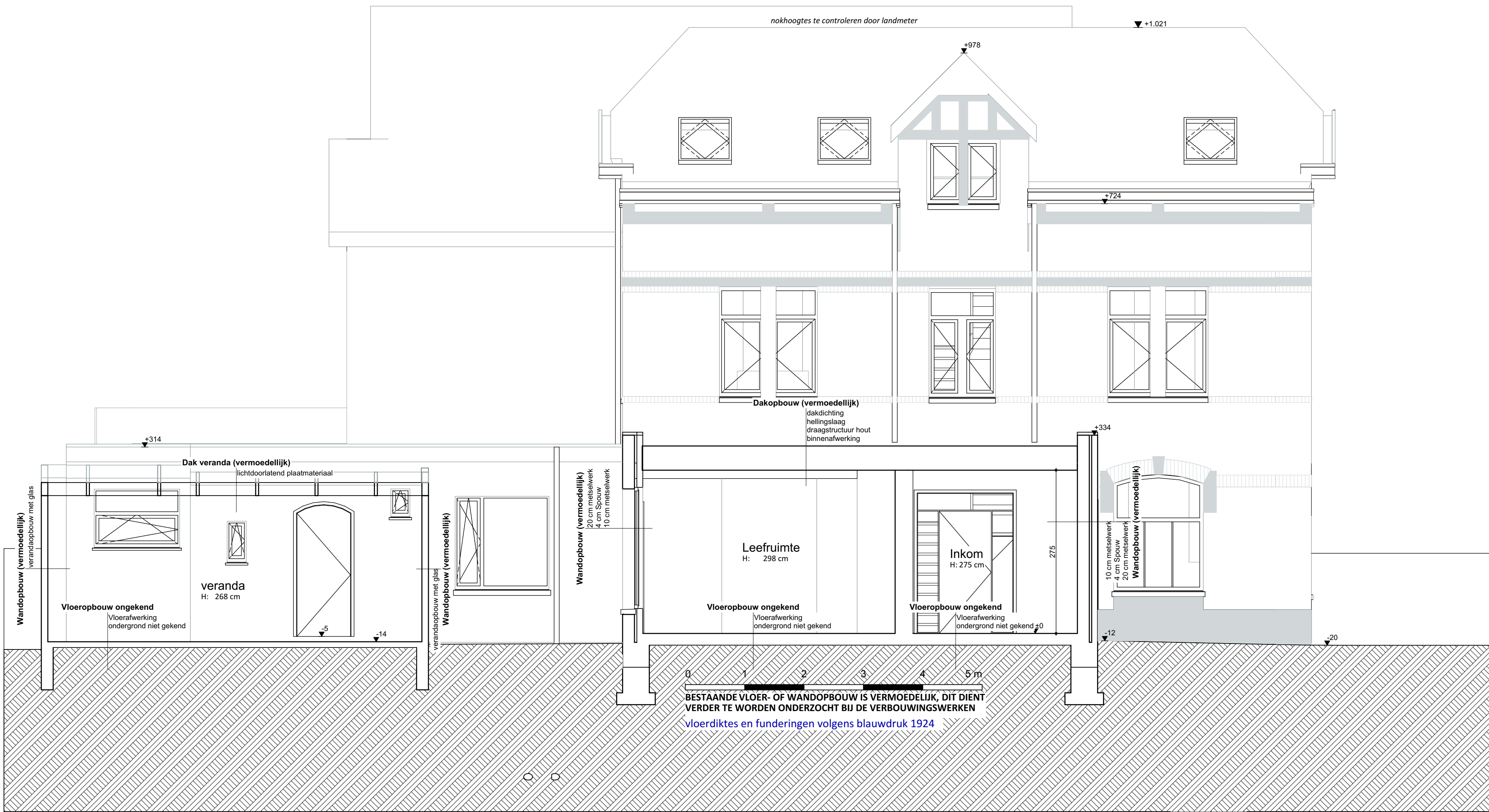
DOORSNEDE S3 - Bestaande toestand
