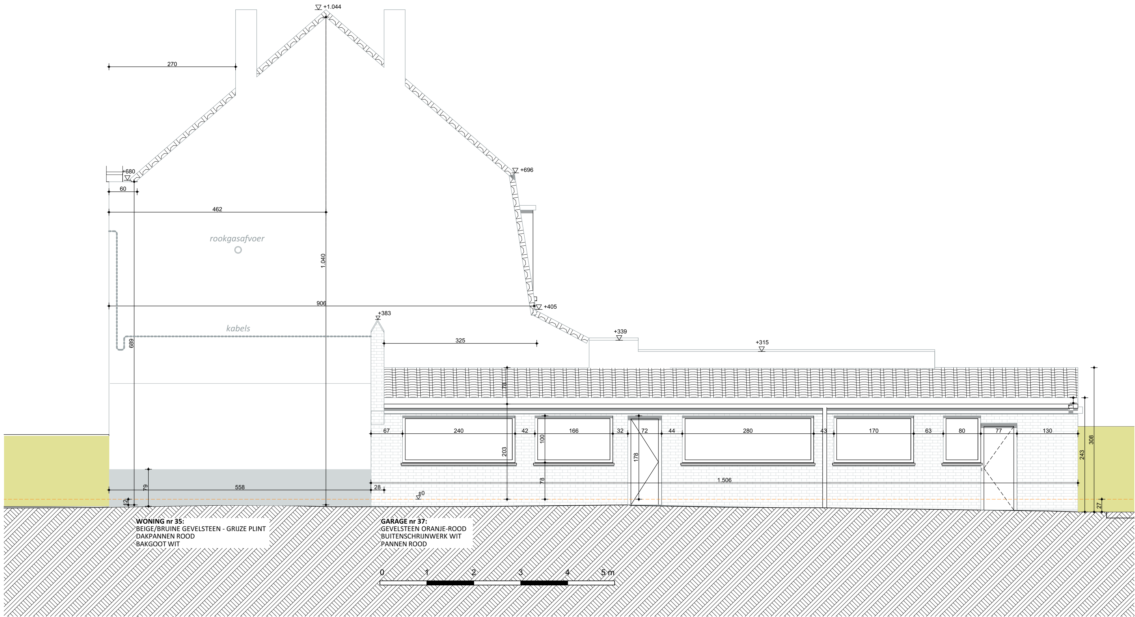
RECHTERGEVEL 2 - Bestaande toestand
