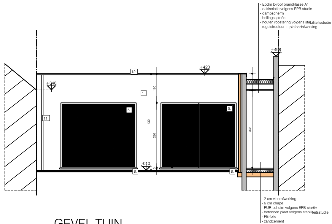
GEVEL TUIN NIEUWE TOESTAND 1/100
