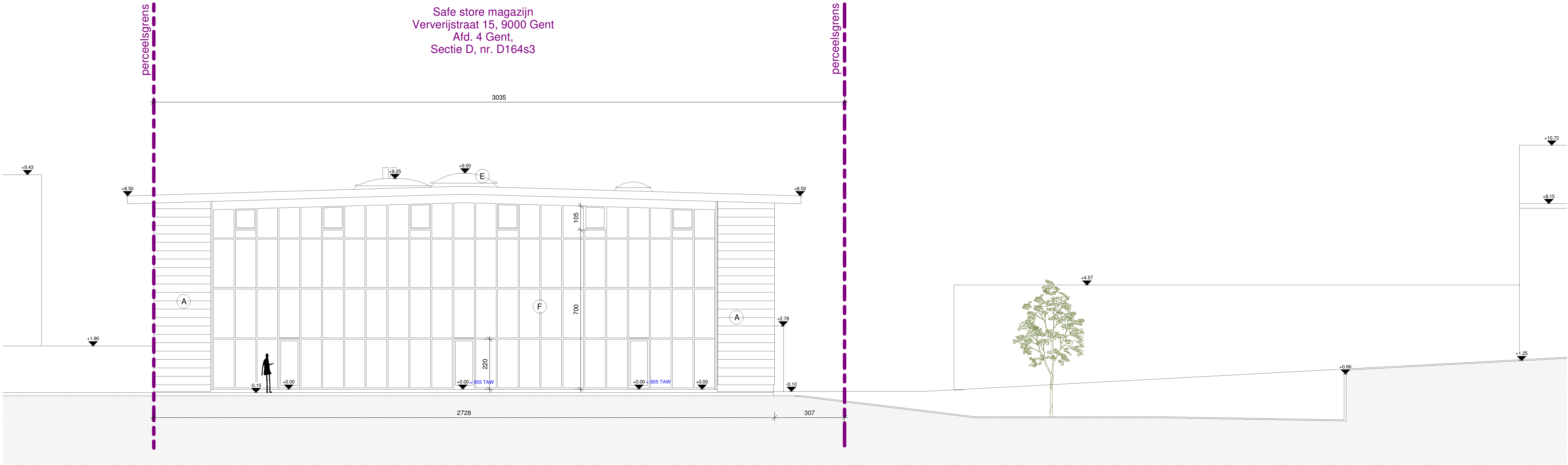
1 1 : 100 Linkergevel vergunde toestand
