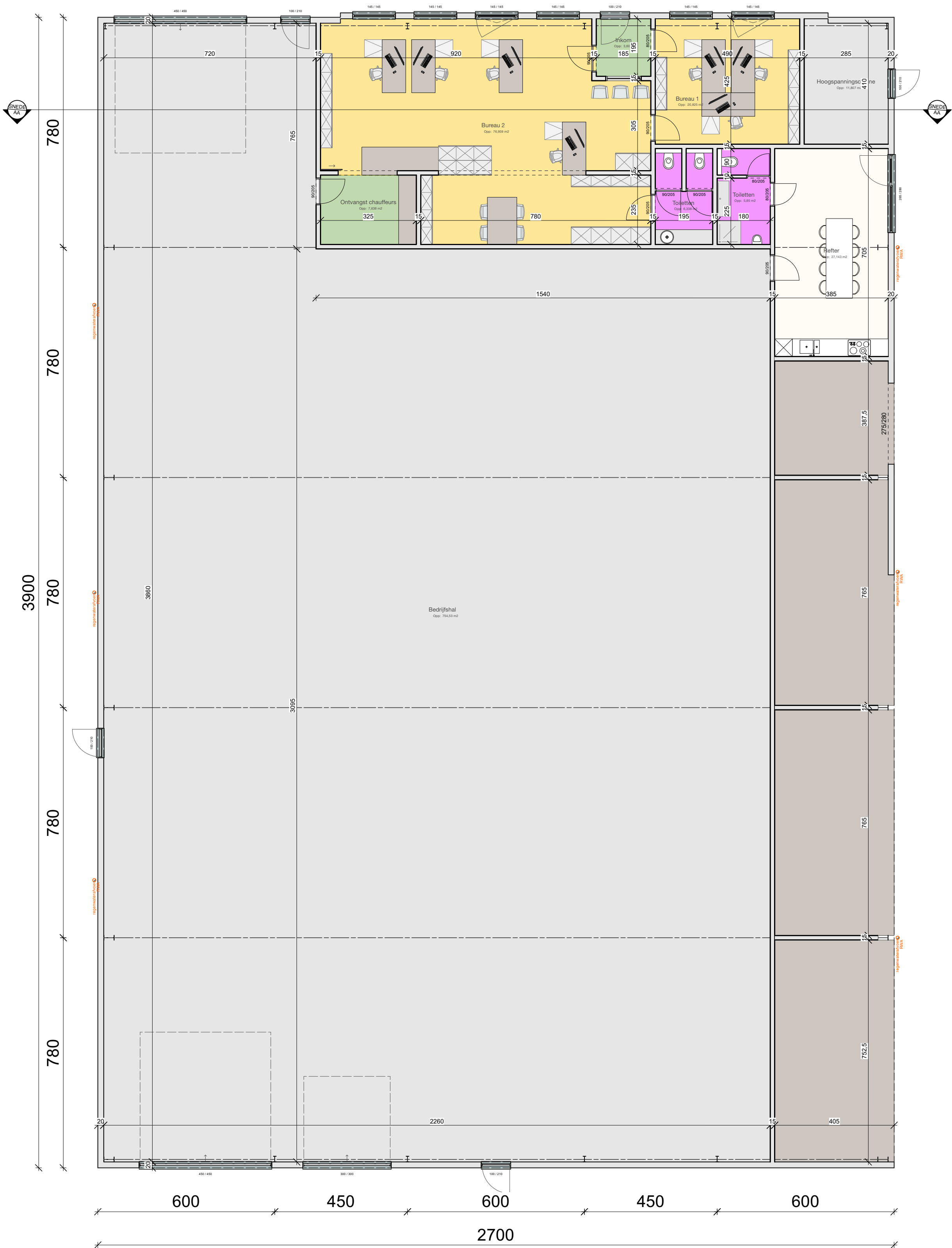
Grondplan bedrijfshal BESTAAND
