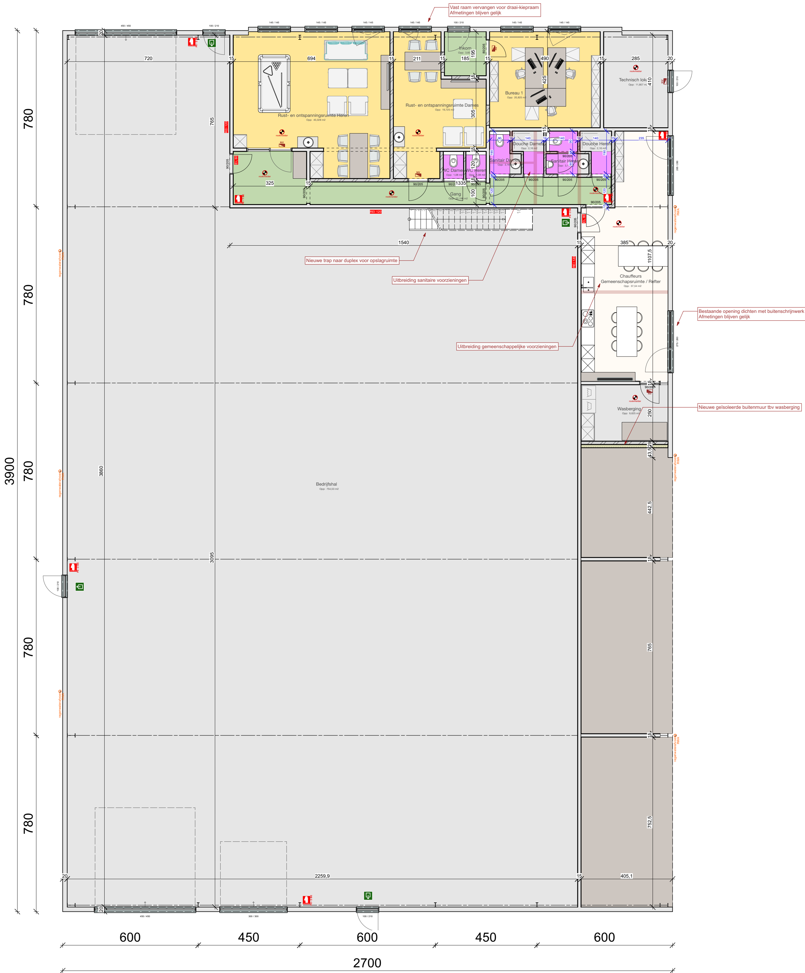
Grondplan bedrijfshal NIEUW
