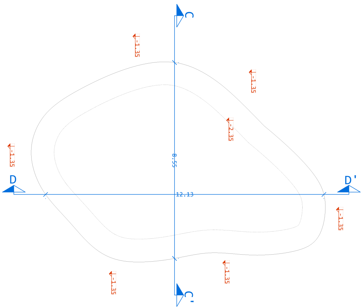
bovenaanzicht wadi
