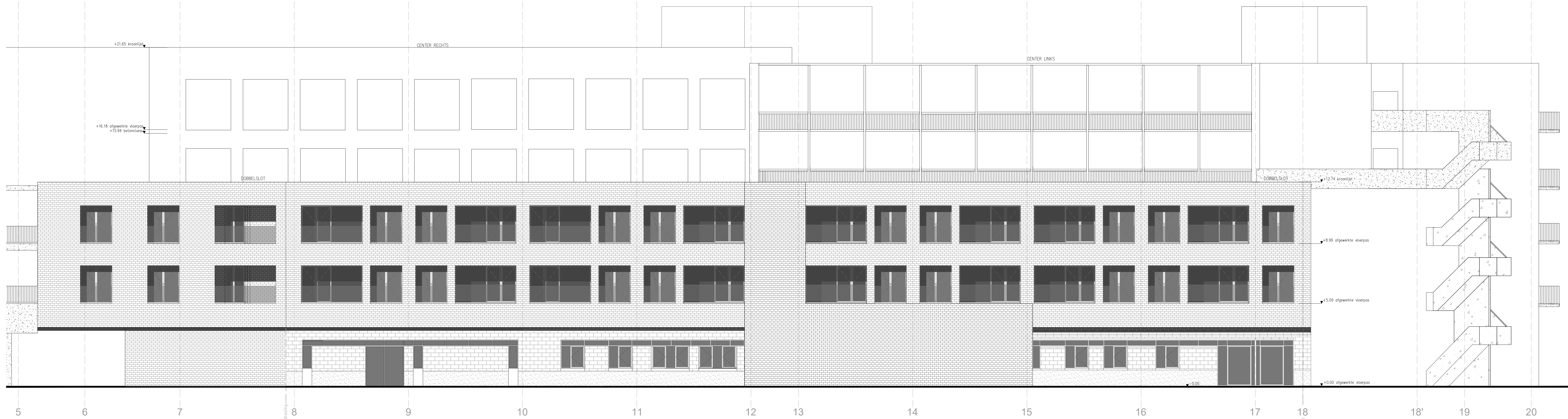
G1 - VOORGEVEL LANGS DOBBELSLOT
