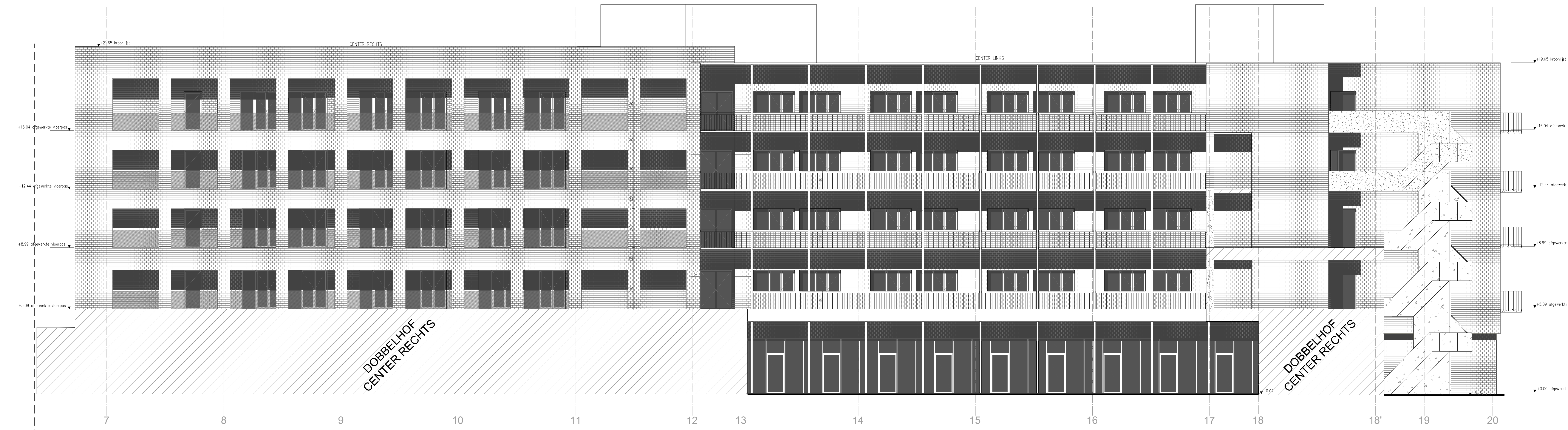
G1 - BINNENGEVEL CENTER RECHTS - CENTER LINKS (Dobbelhof)
