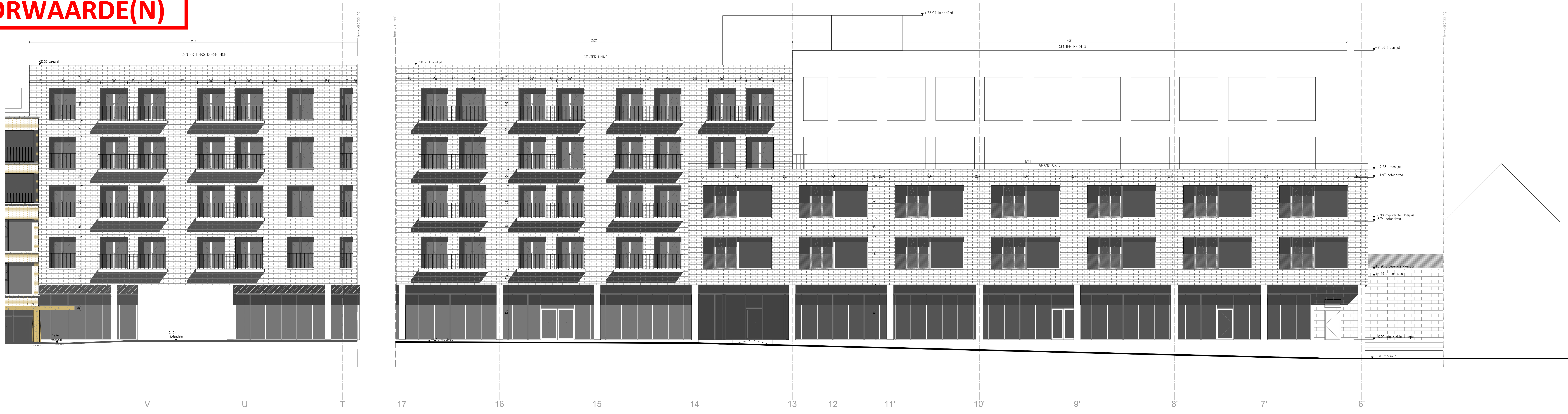
G1 - GEVEL CENTER LINKS MIDDENPLEIN
