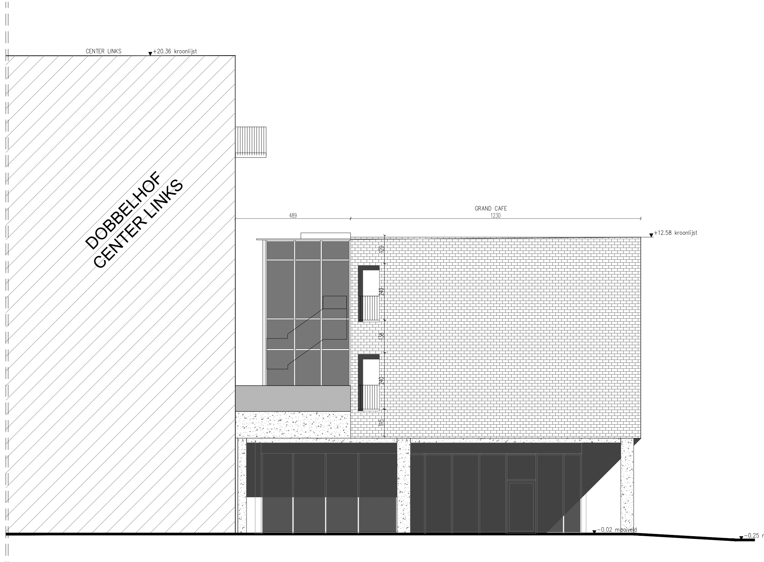
G4 - ZIJGEVEL LINKS GRAND CAFE
