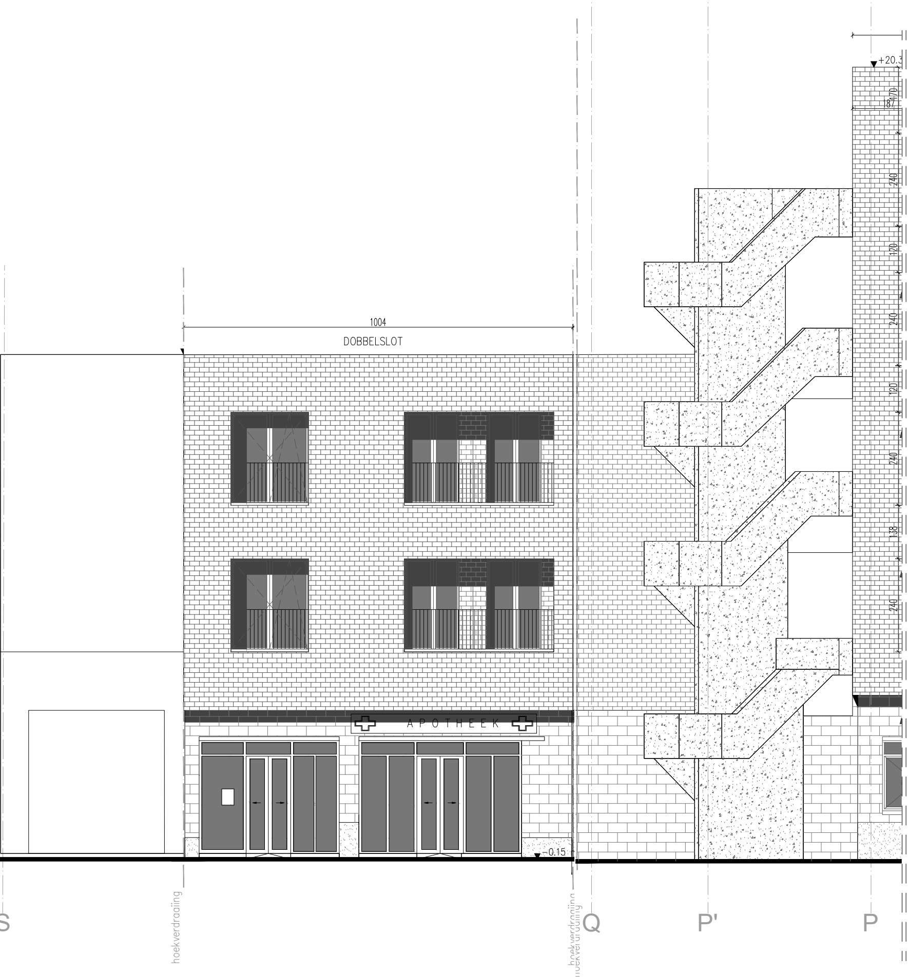
G3 - ZIJGEVEL - SCHUINE GEVEL
