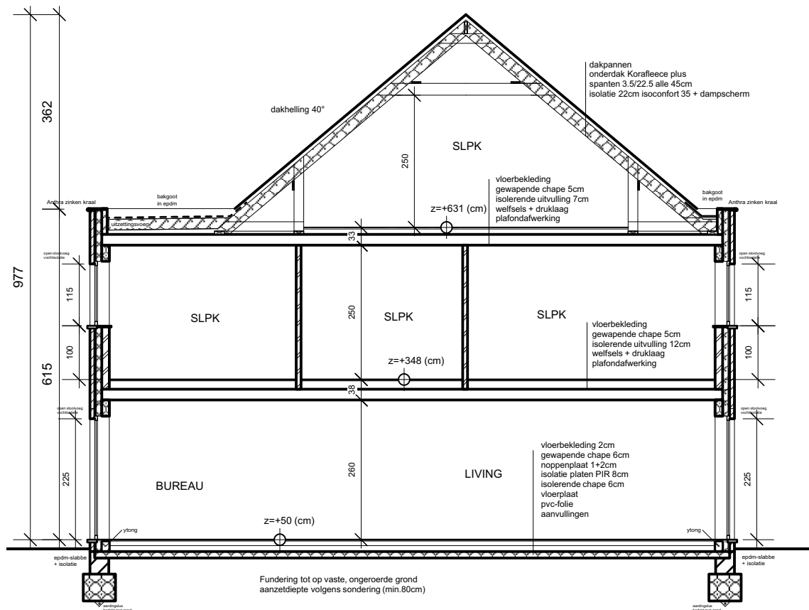
DOORSNEDE A-A 1/100
