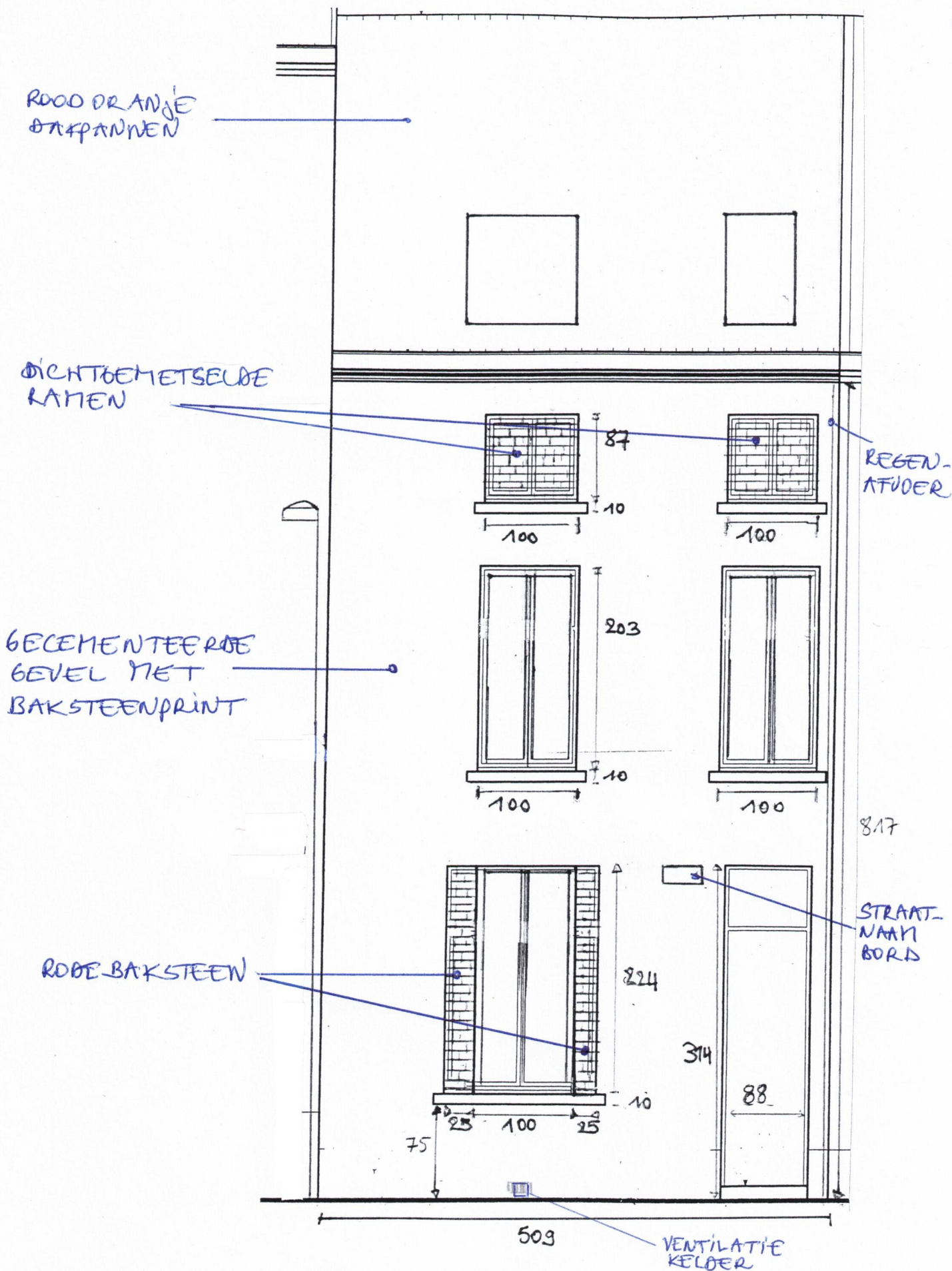
BESTAANDE GEVEL (schaal 1/50)
