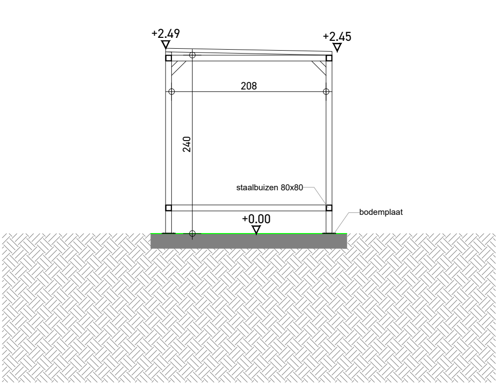
Snede BB
