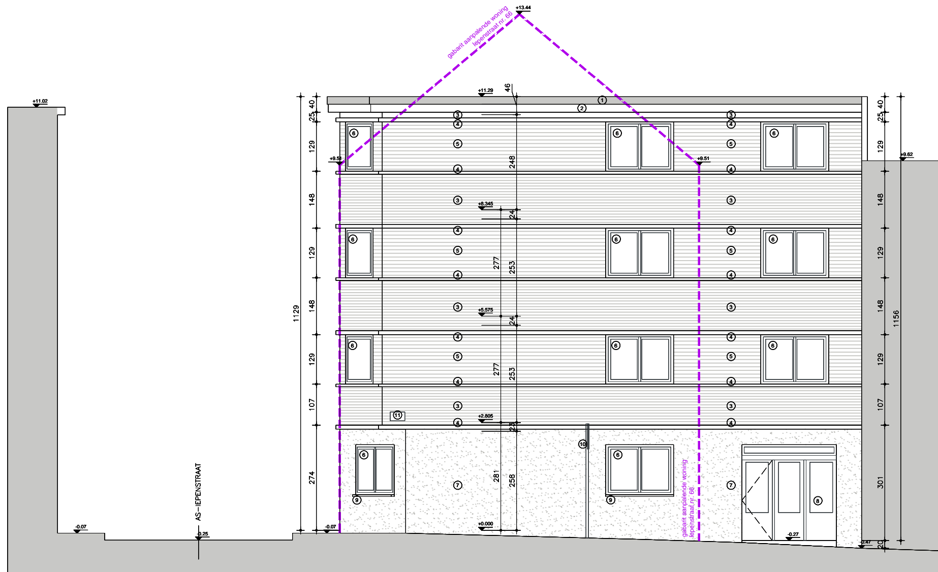
GEVEL KARENSTRAAT
