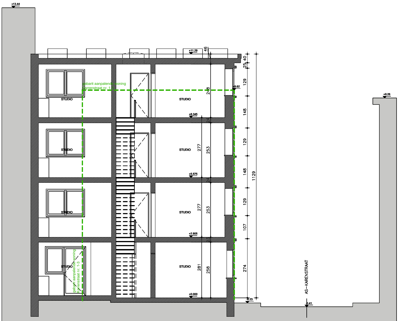
DOORSNEDE - 01
