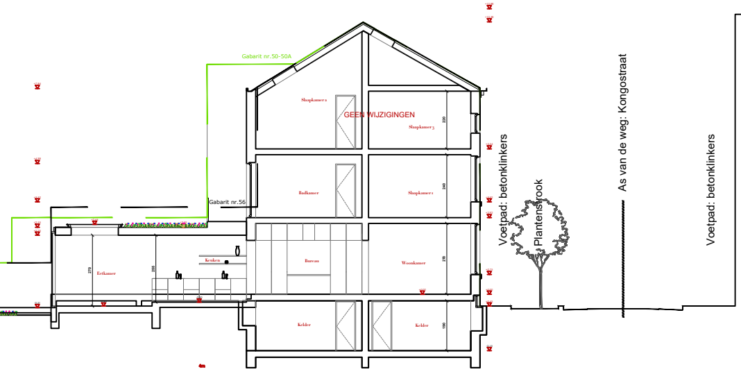
TERREINSNEDE A-A'- VERGUNDE TOESTAND
