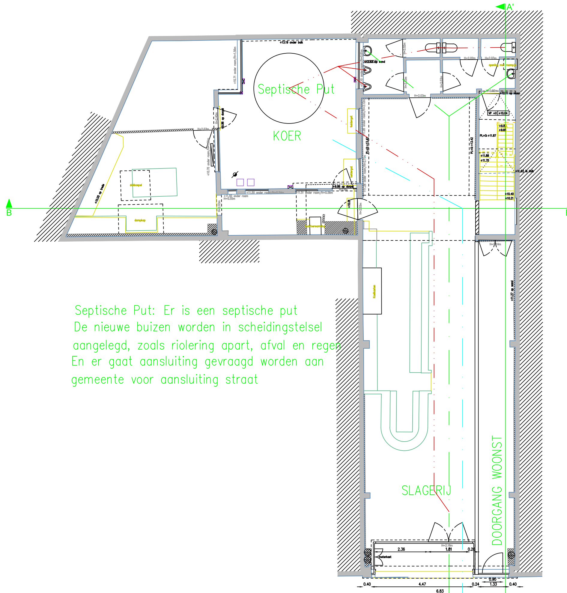
Nieuwe toestand RIOLERINGSPLAN Schaal 1/100
