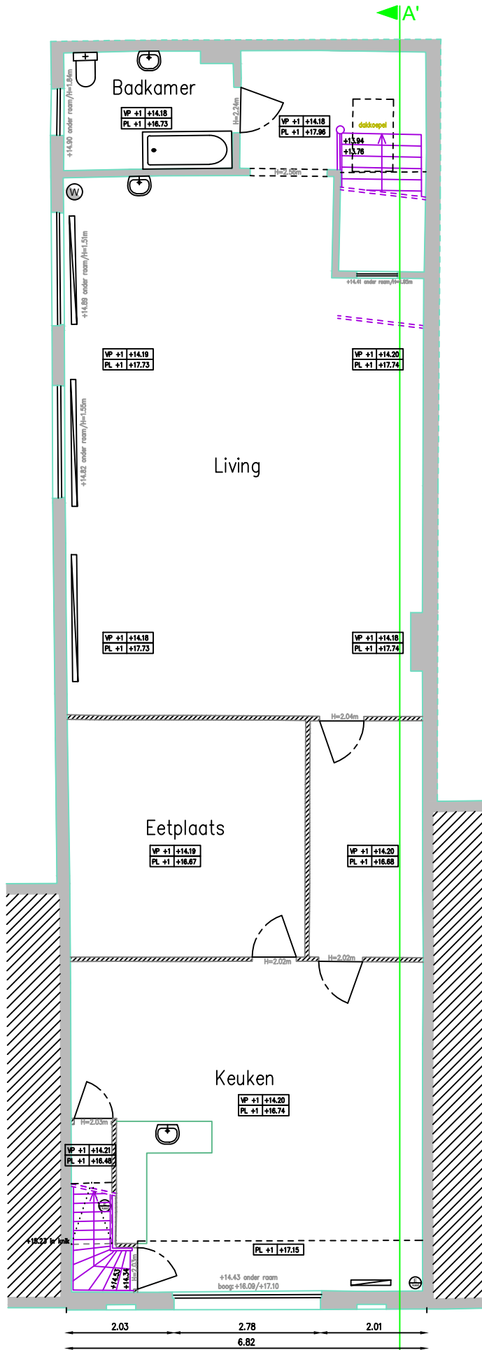
Bestaande toestand Eerste Verdieping Schaal 1/100
