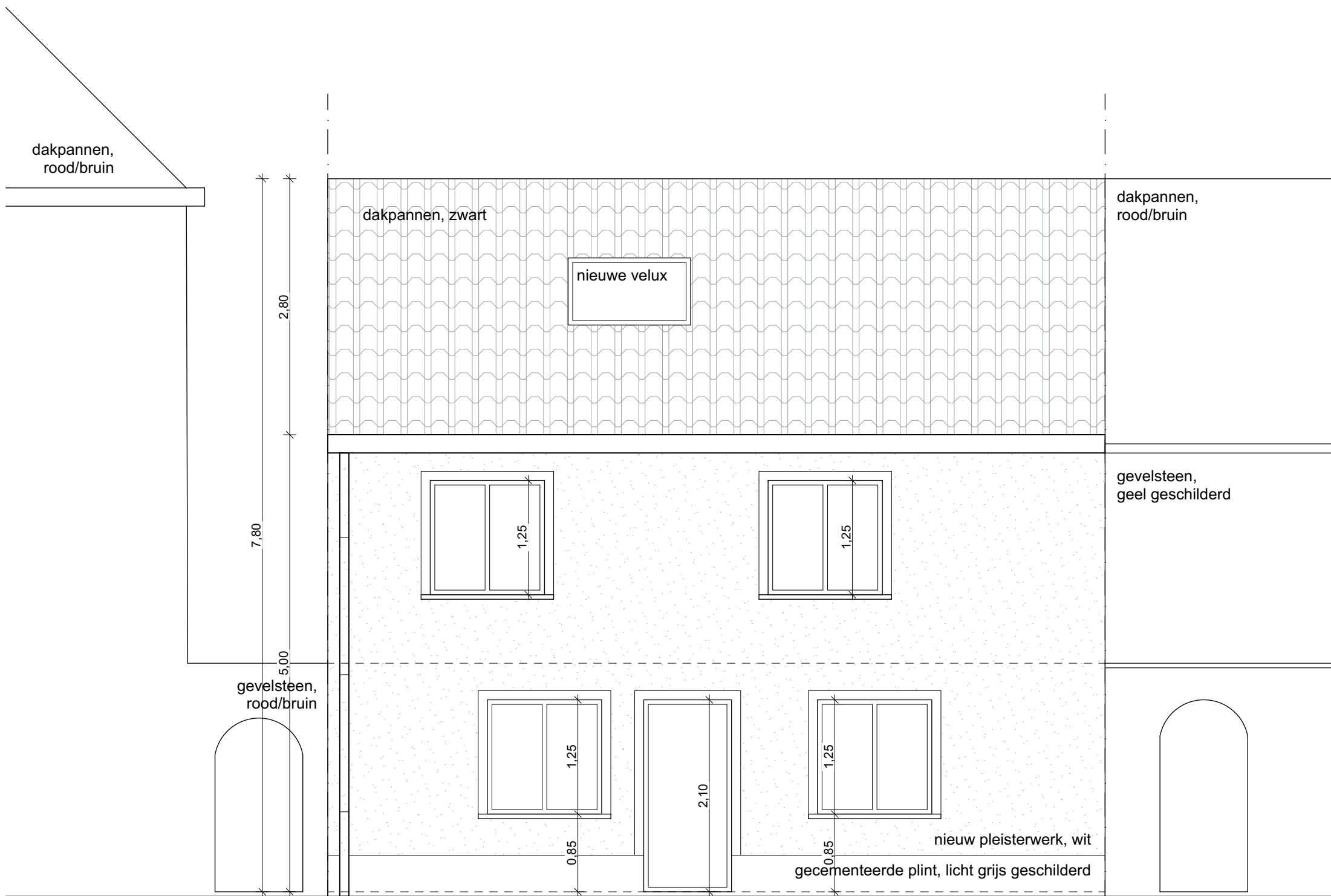
STRAATGEVEL, nieuwe toestand schaal 1/50, maataanduiding in meter.
