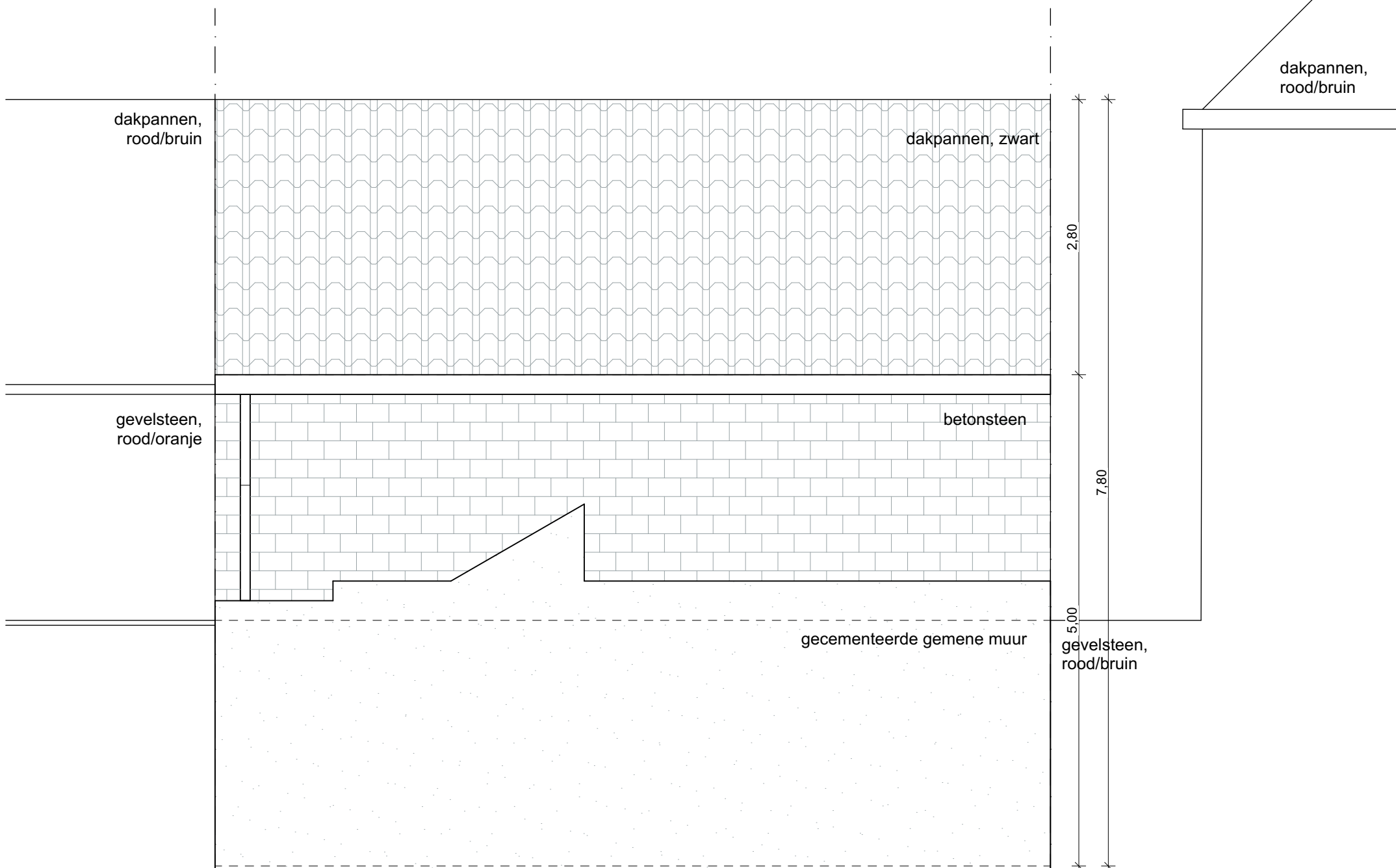
TUINGEVEL, bestaande toestand schaal 1/50, maataanduiding in meter.
