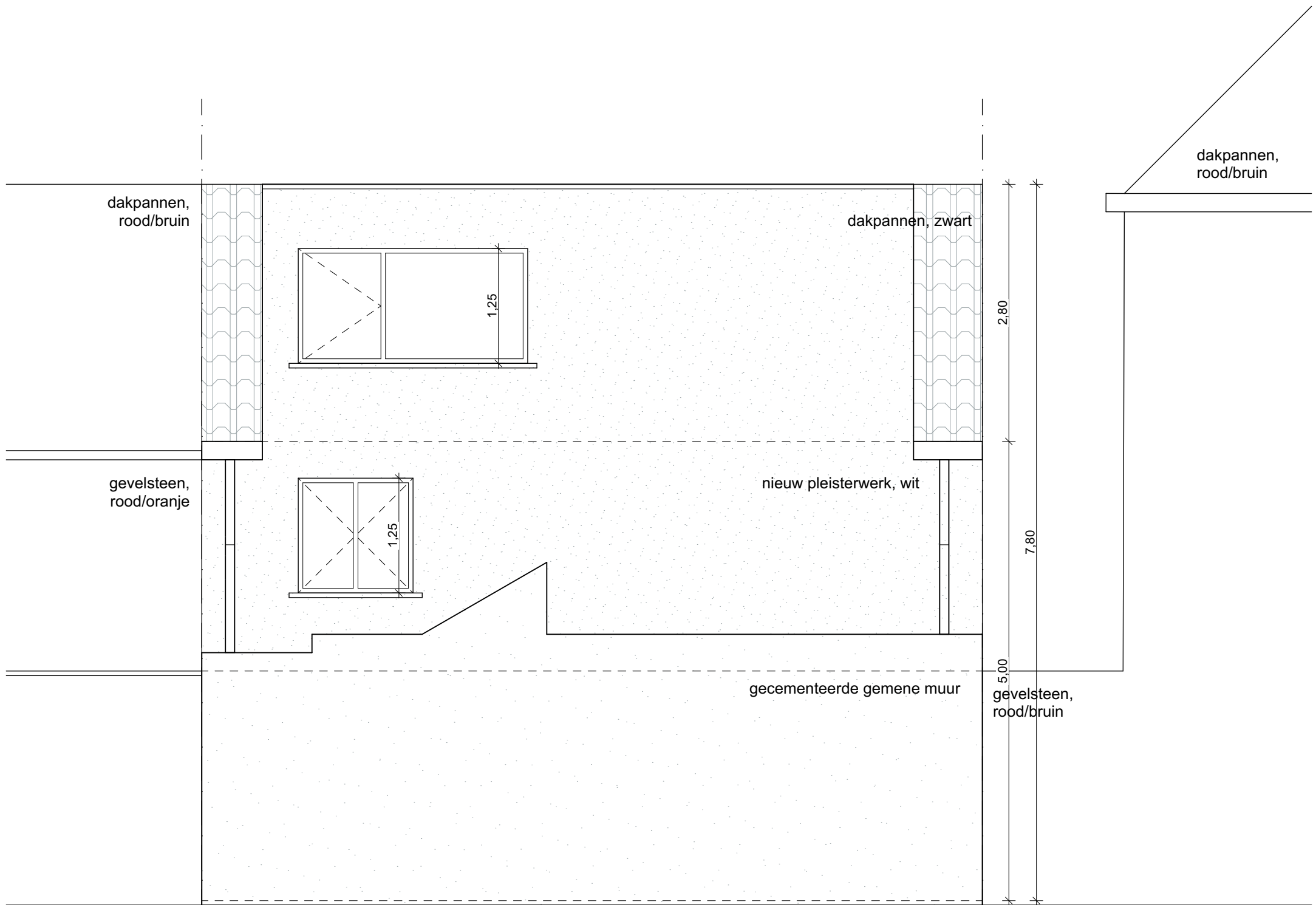
TUINGEVEL, nieuwe toestand schaal 1/50, maataanduiding in meter.
