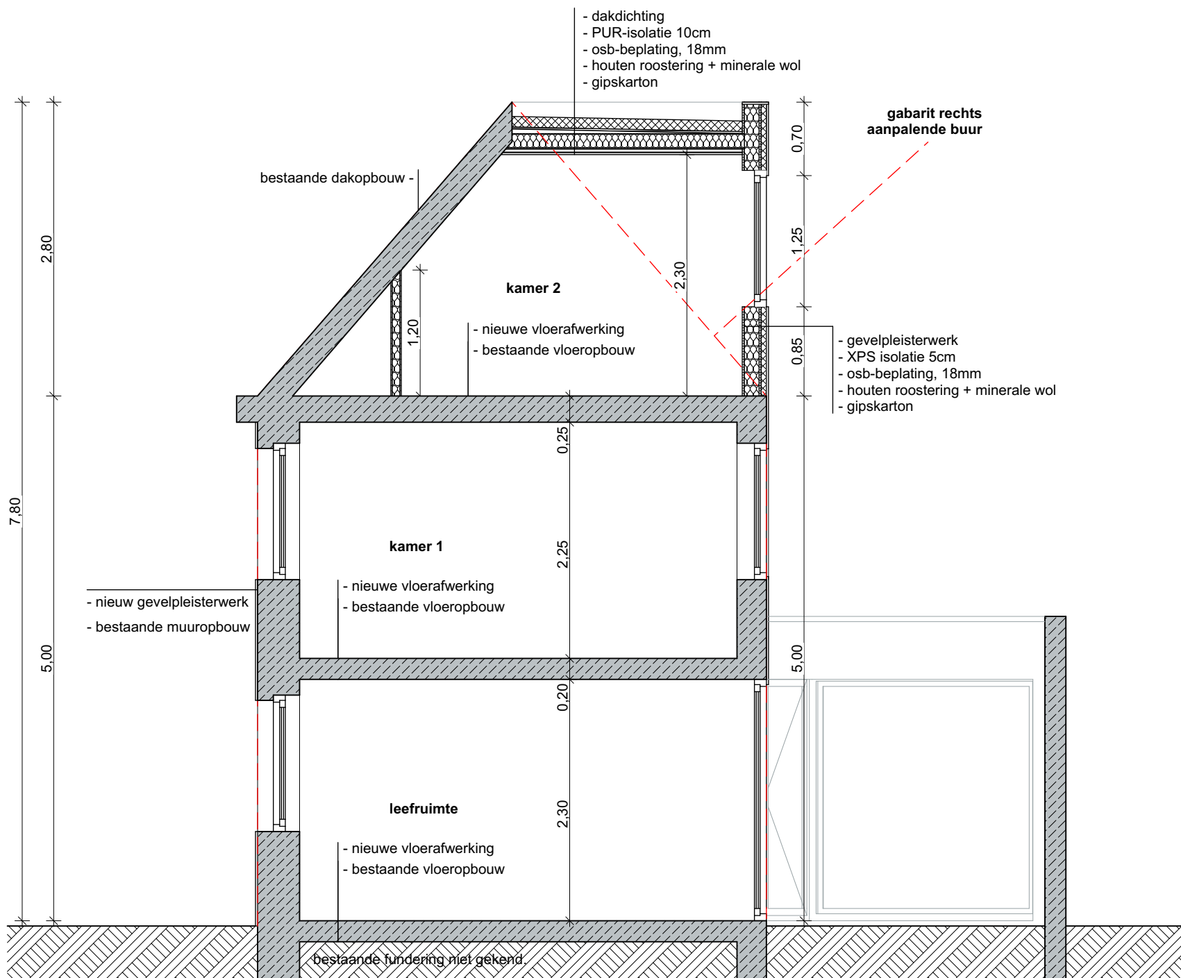
DOORSNEDE AA, nieuwe toestand schaal 1/50, maataanduiding in meter.
