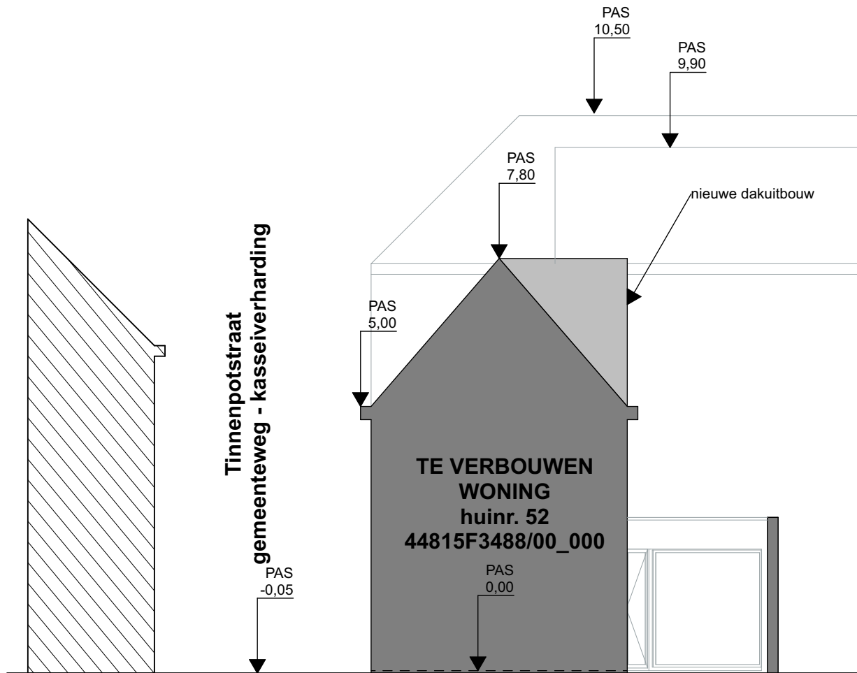
TERREINPROFIELSNEDE, nieuwe toestand schaal 1/100, maataanduiding in meter.
