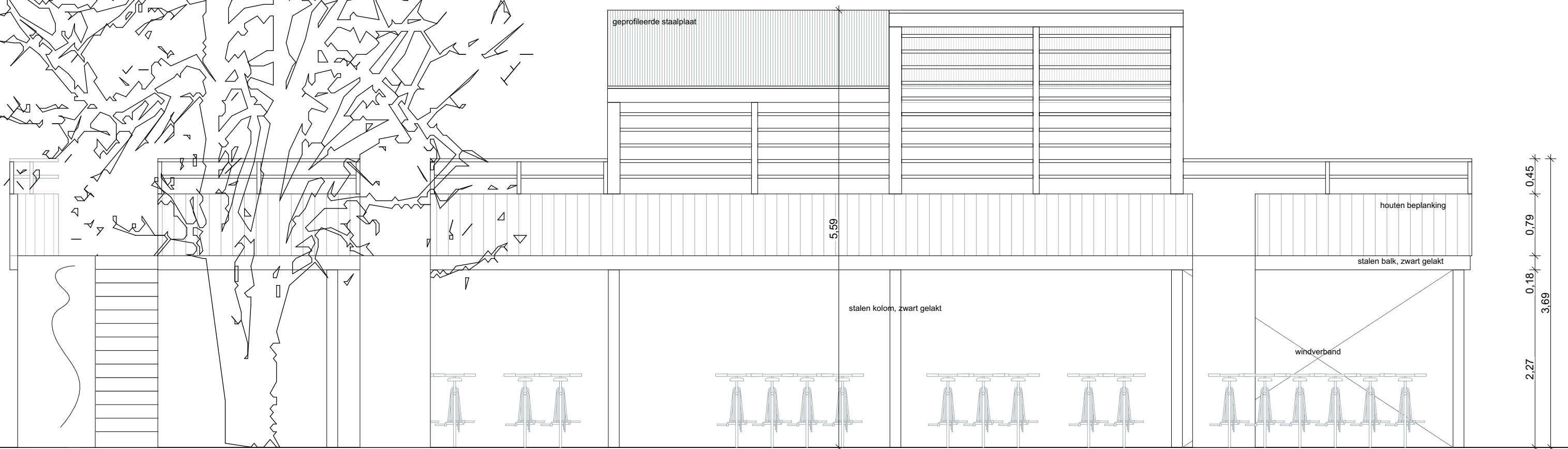
GEVEL 3 schaal 1/50, maataanduiding in meter.
