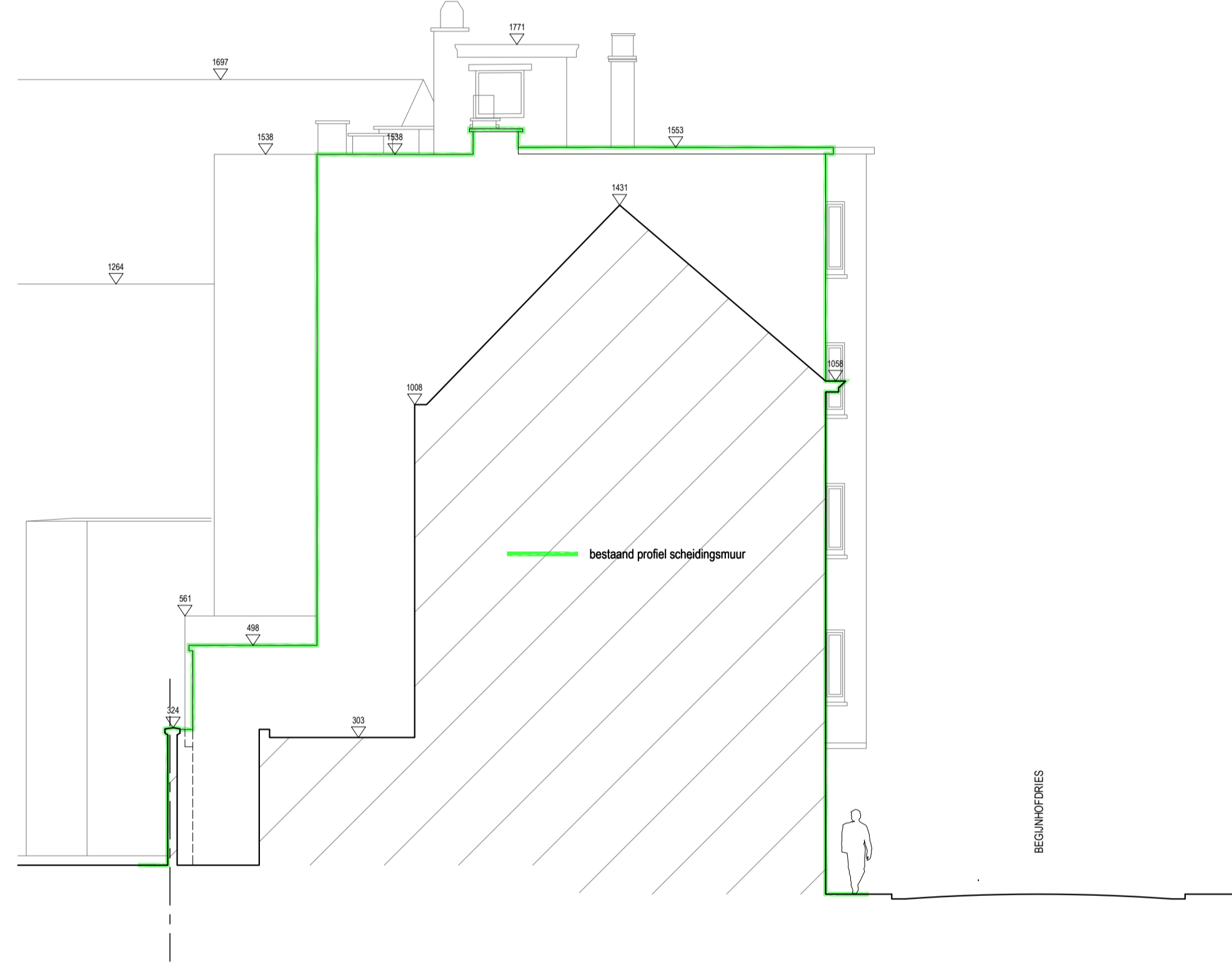
TERREINPROFIEL LINKERBUUR bestand
